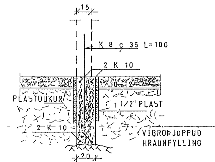
SNID Í INNVEGG 1:20
