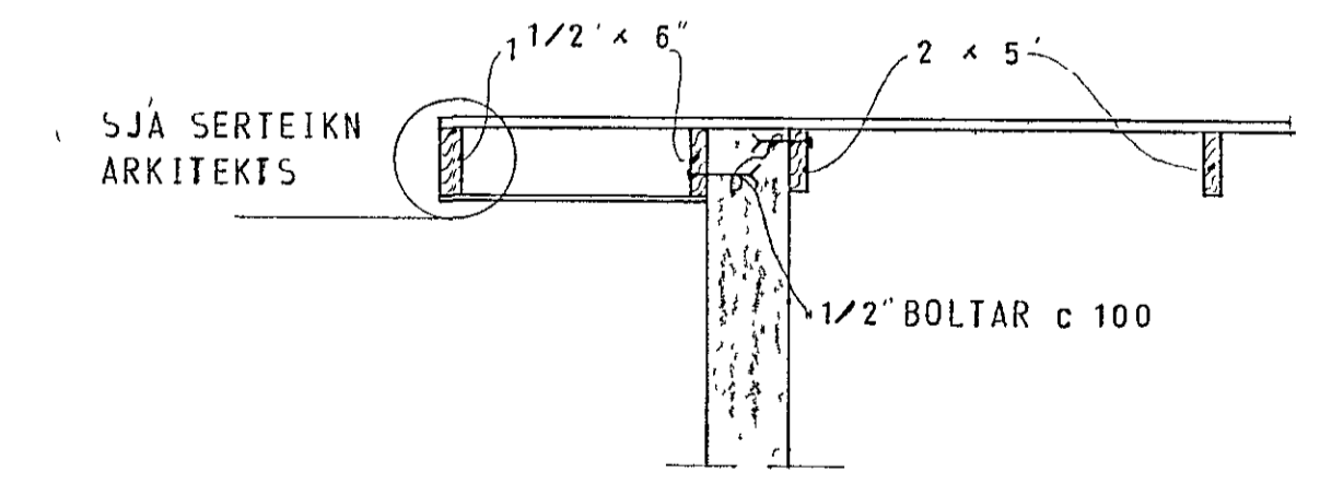
SNID D 1:20
