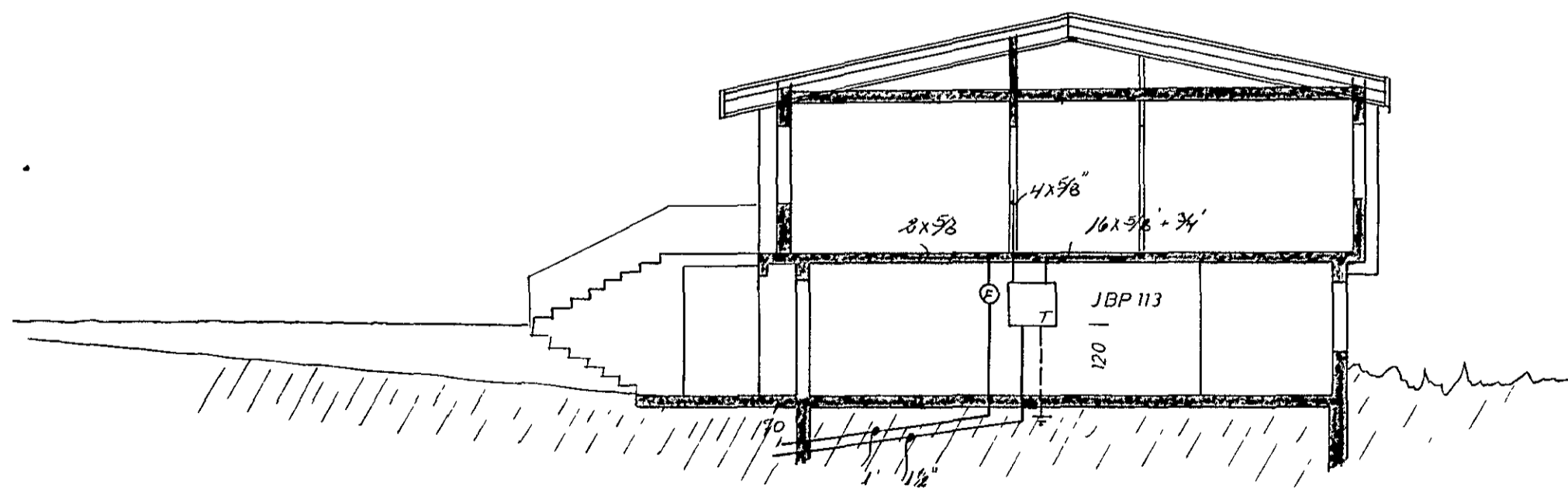
snid A-A 1 100
