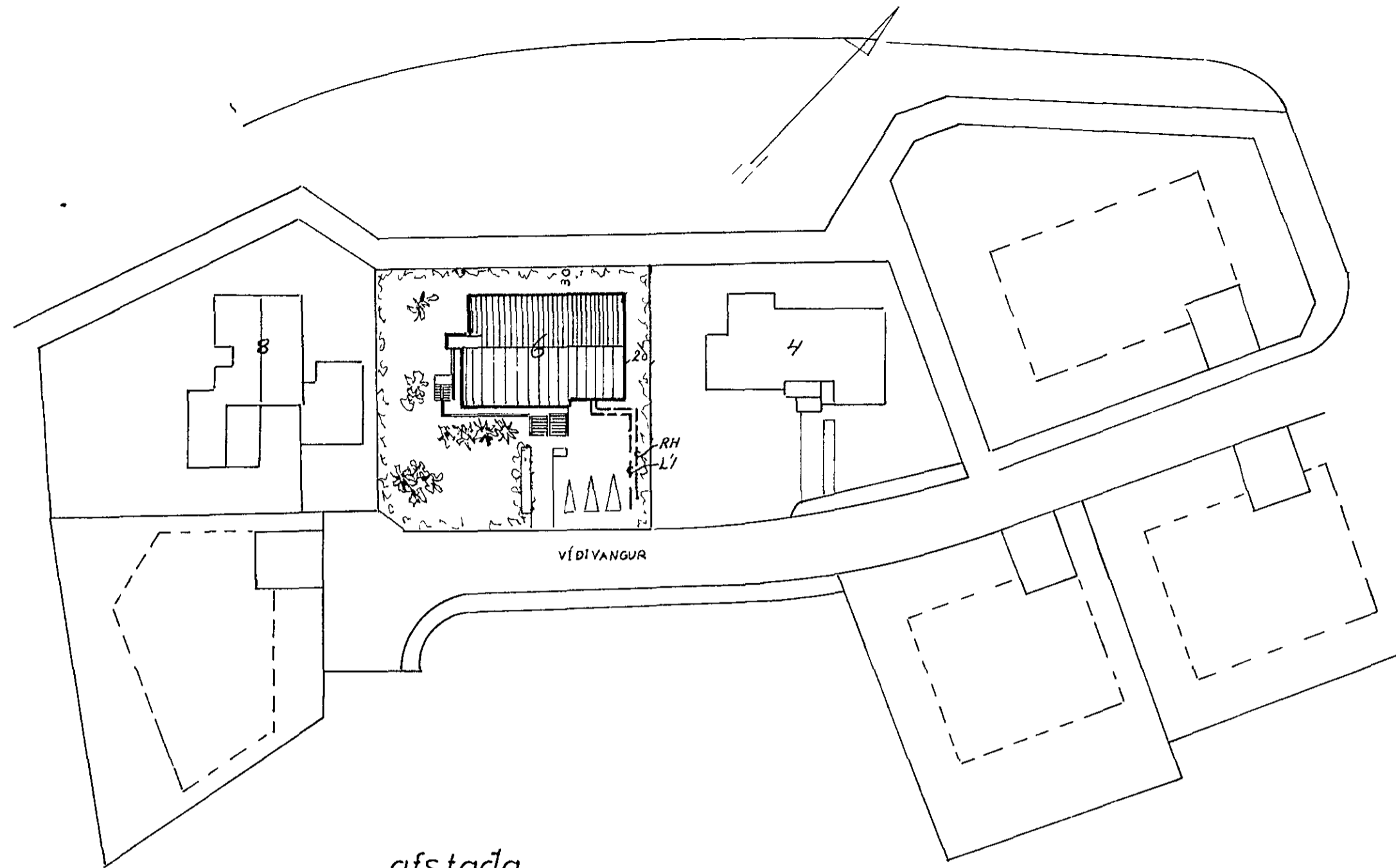
afstada 1 500
