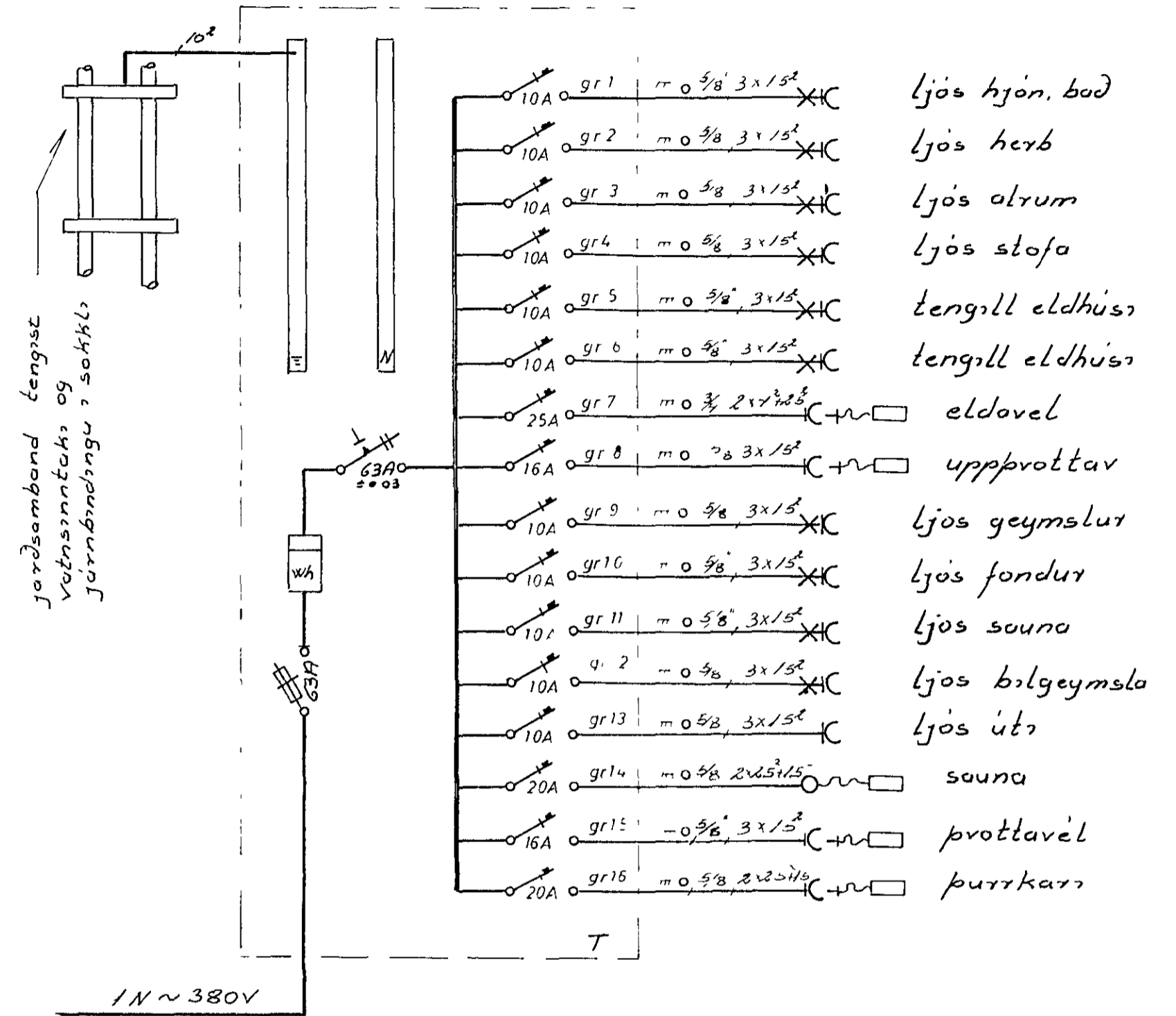
einlinumynd
