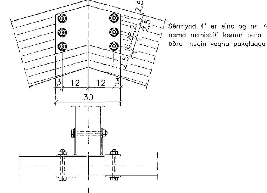
Sérmynd 4'. 1:10
