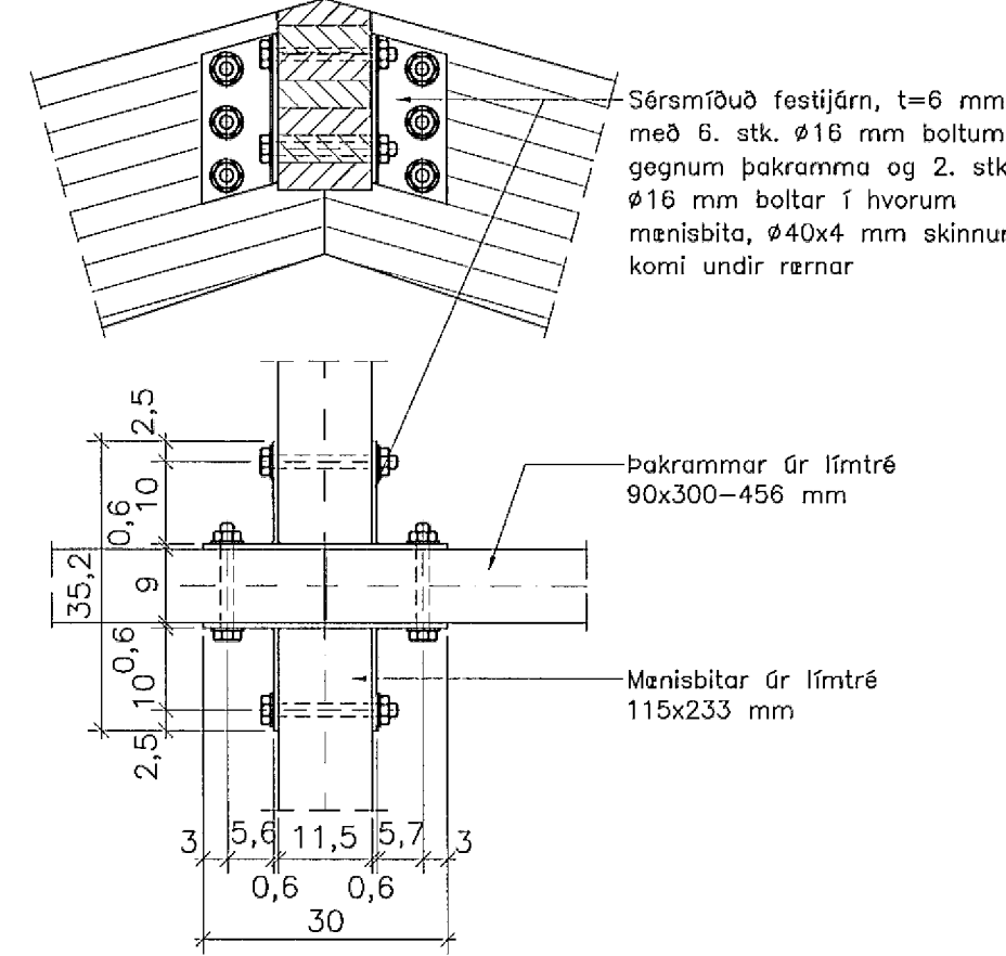
Sérmynd 4. 1:10
