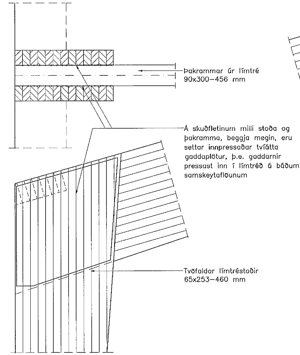
Sérmynd 2. 1:10
