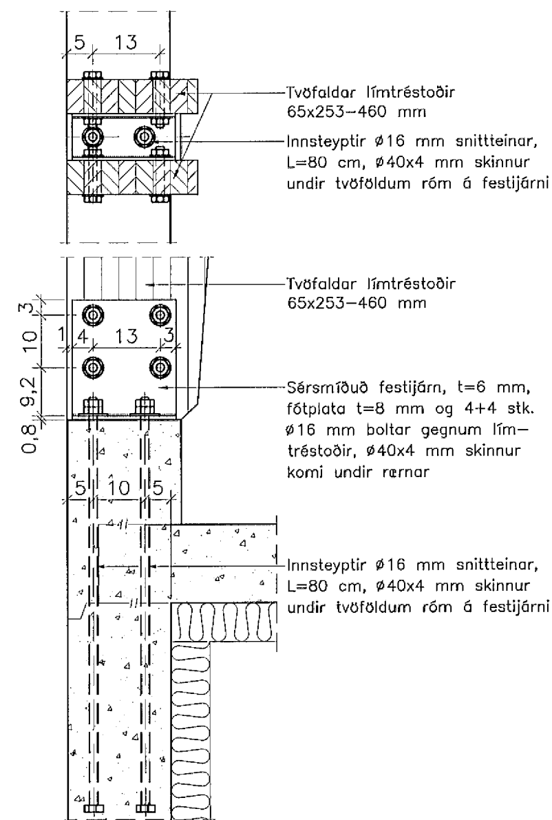
Sérmynd 1. 1:10
