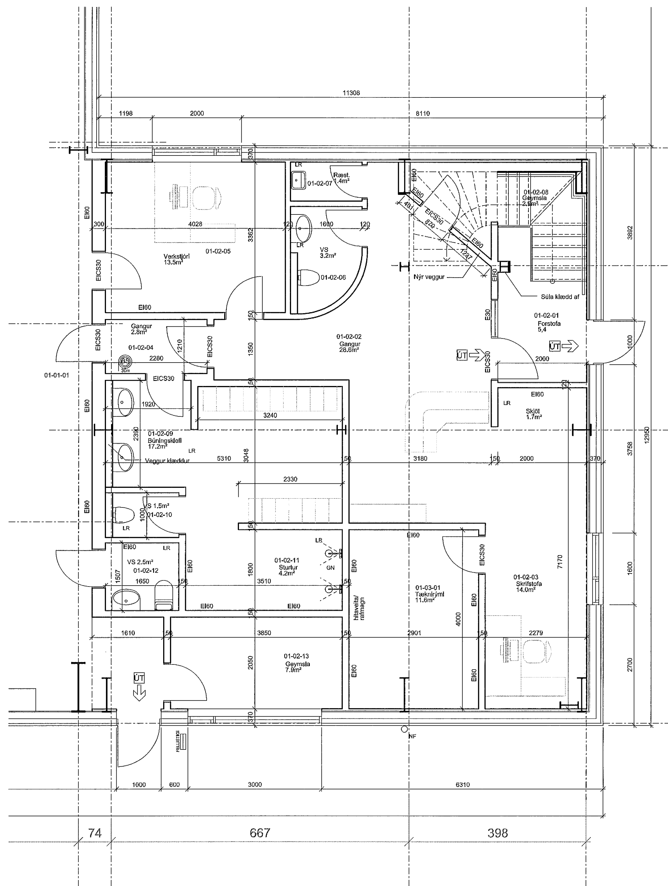
1 GRUNNMYND 1:50 Grunnmynd 1. Hæðar
