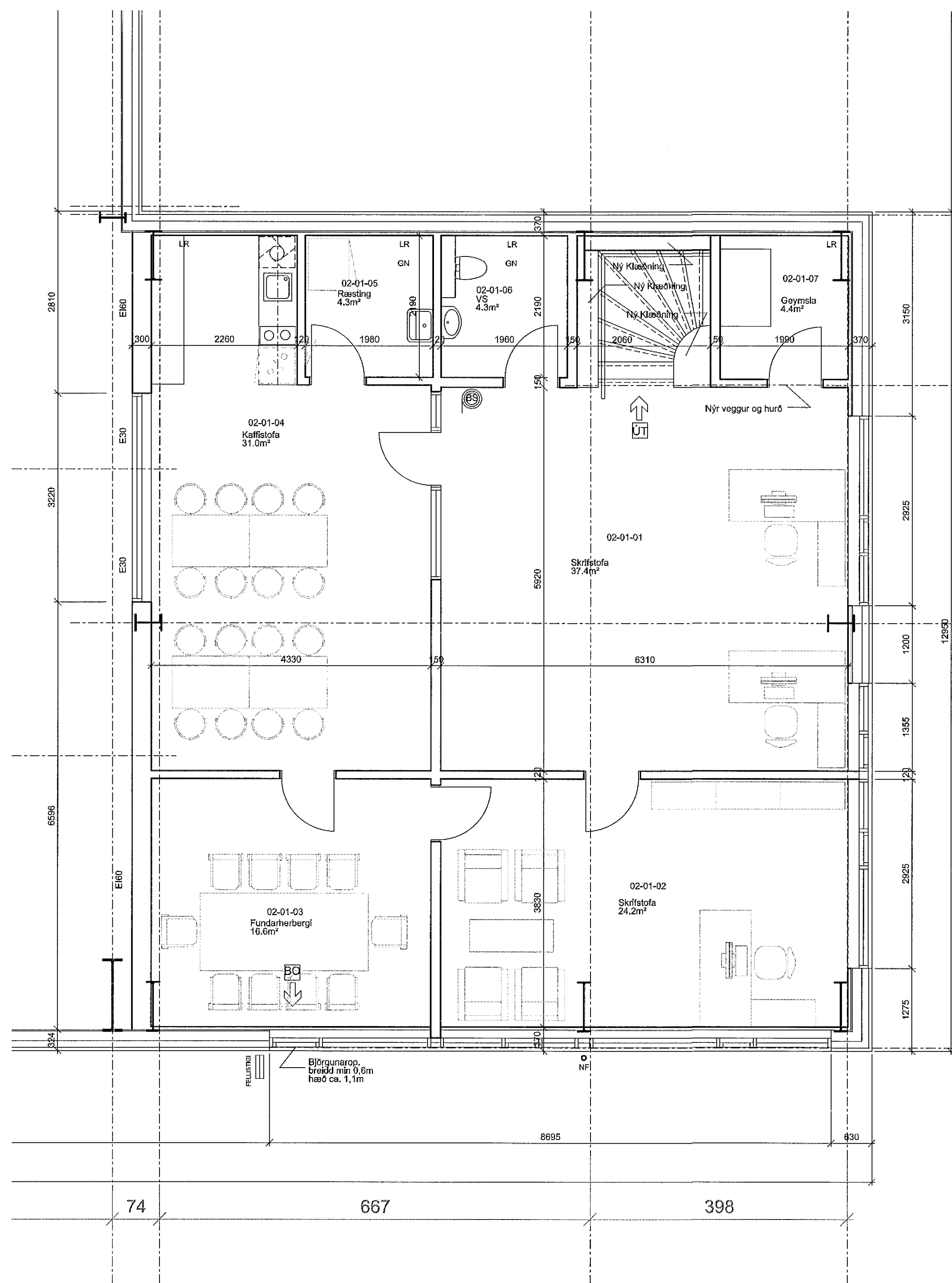
2 GRUNNMYND 1:50 Grunnmynd 1. Hæðar
