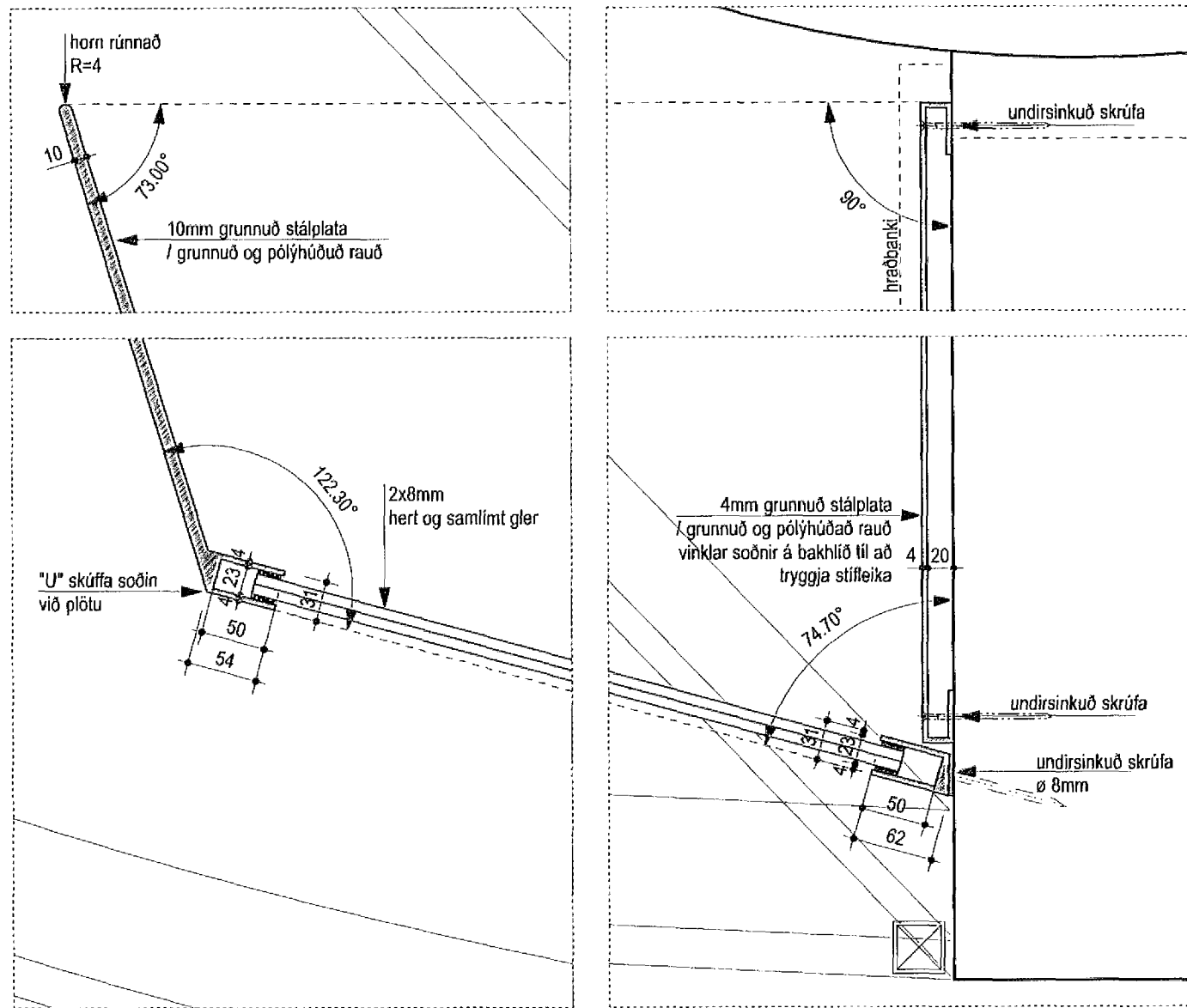
1 DEILI mkv: 1:5
