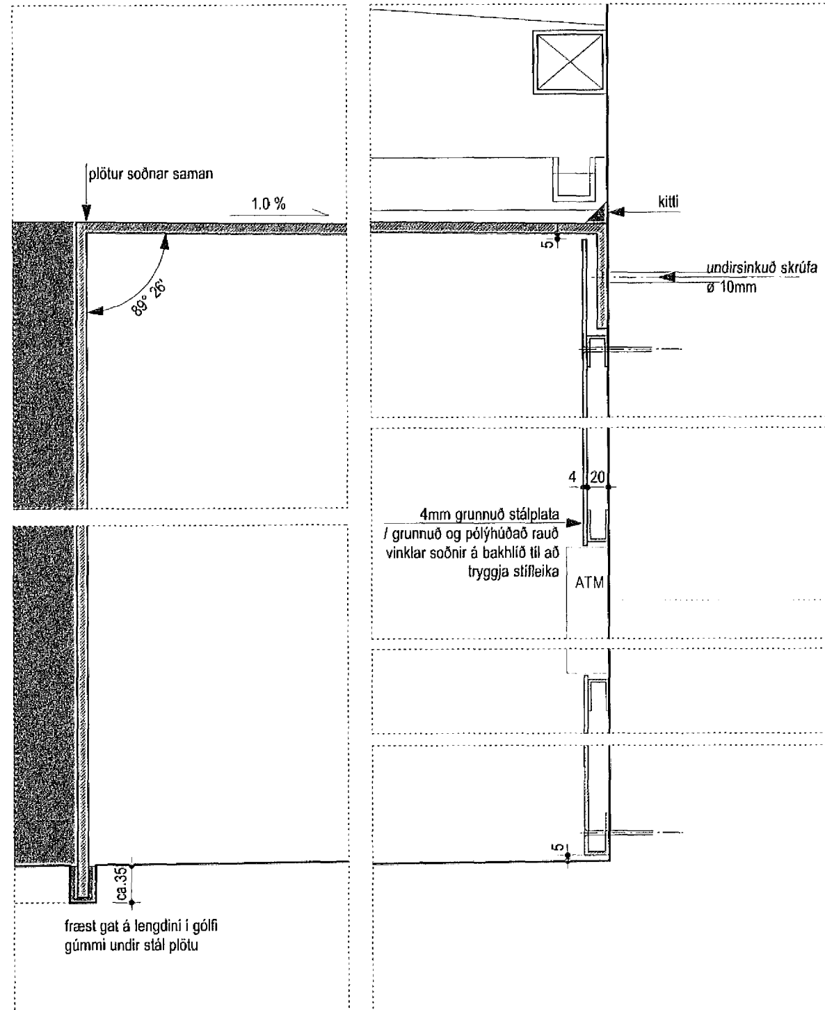
2 DEILI mkv: 1:5
