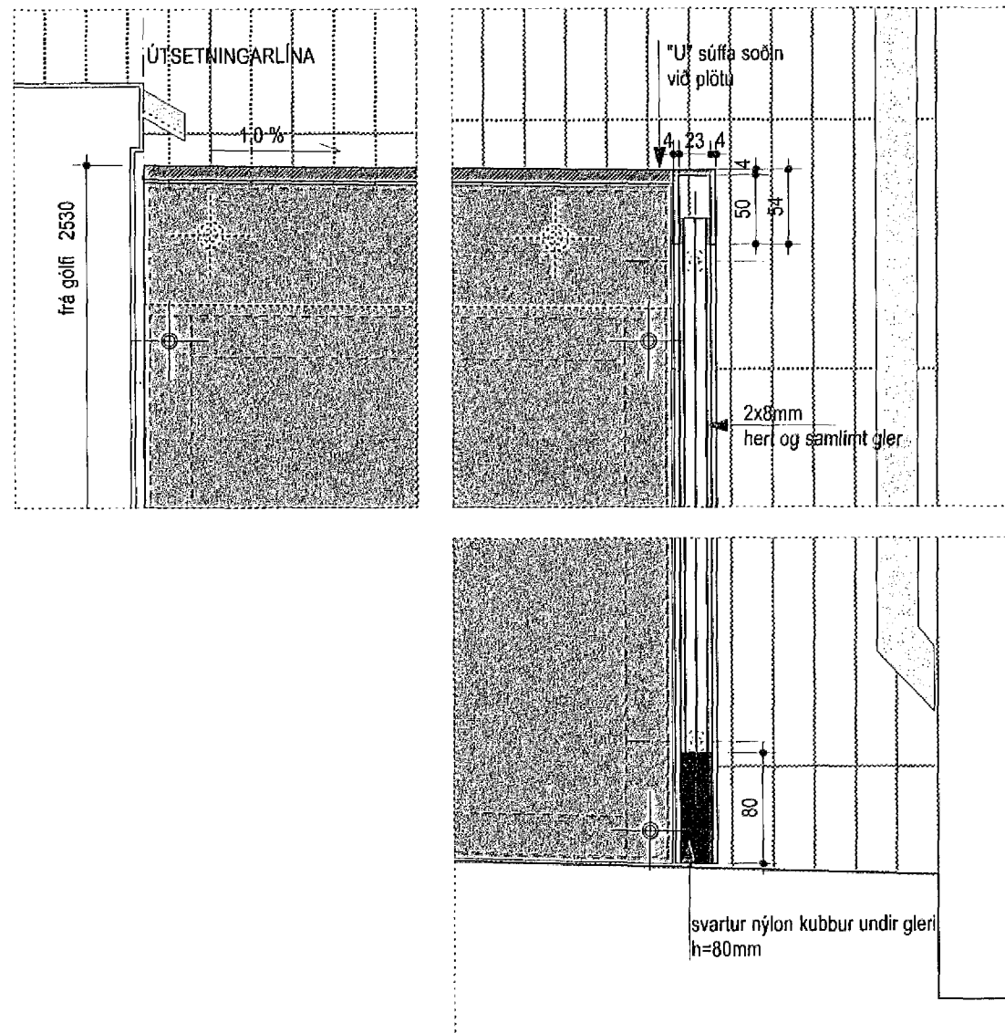
3 DEILI mkv: 1:5
