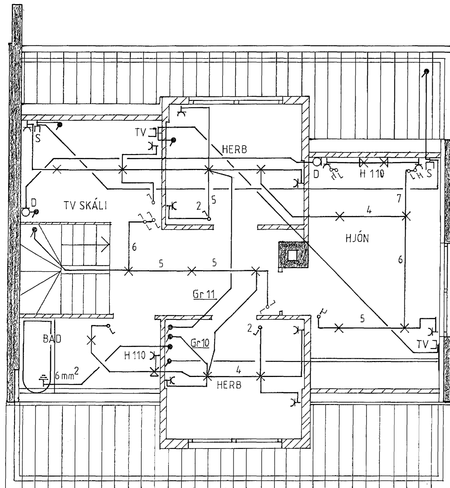
RIS 1:50
