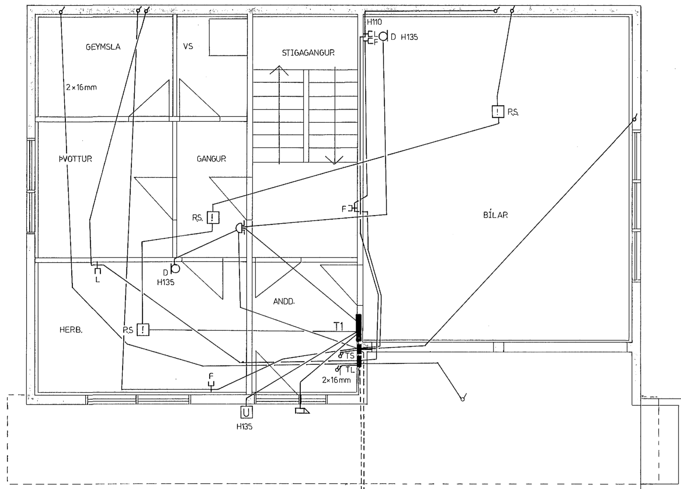
SMÁSPENNA NEDRI HÆÐ M 1:50
