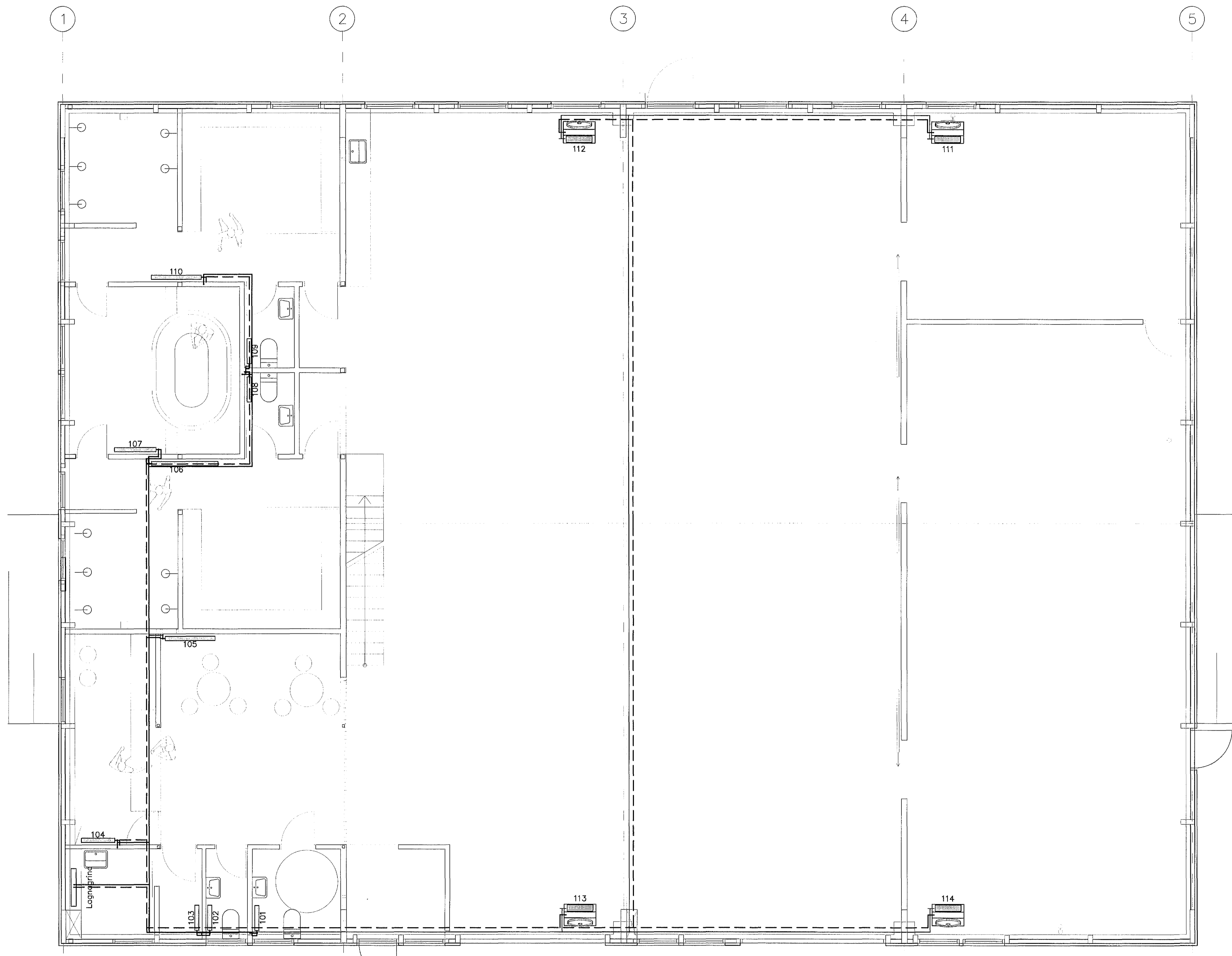
Grunnmynd – Neysluvatn Mkv. 1:50
