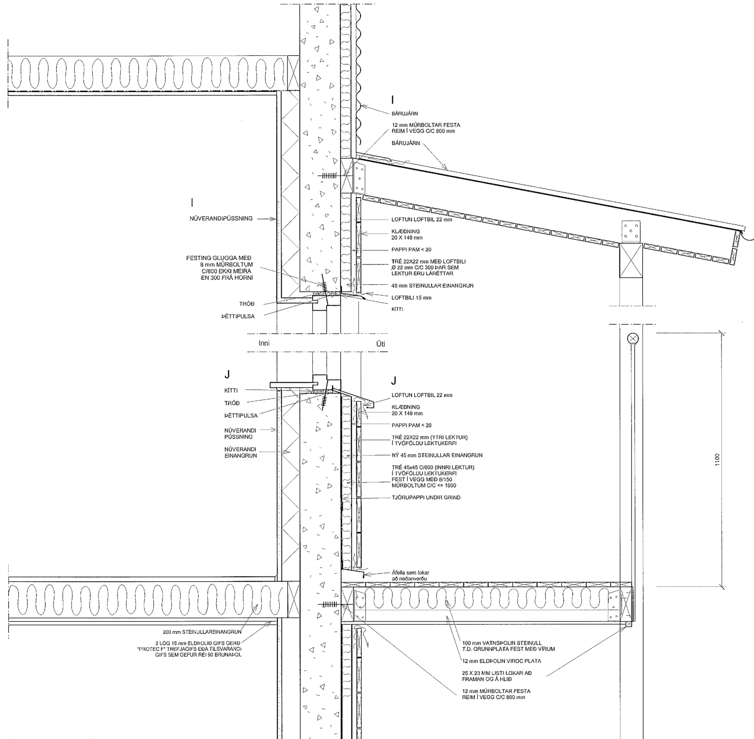
Lóðrett sneiðing í svalagólf og skyggni Mælikvarði 1:10
