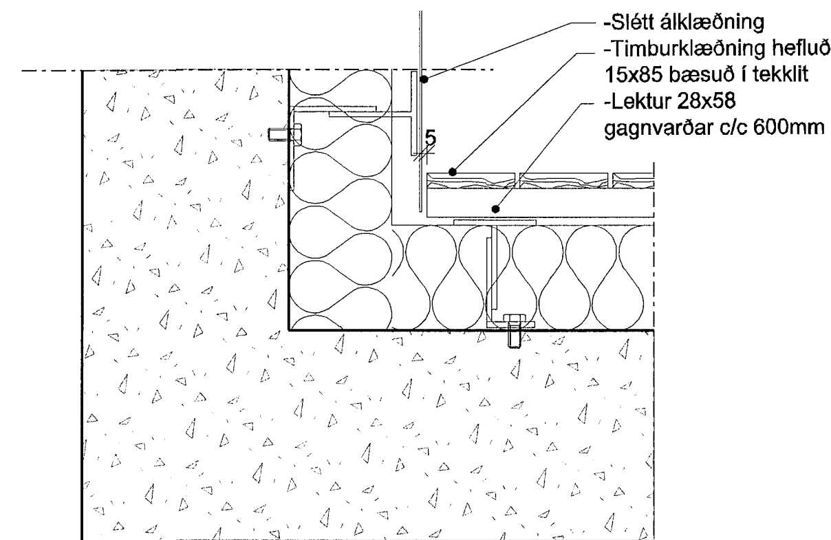
4 DEILI 1:5 INNHORN, SLÉTT/VIÐUR
