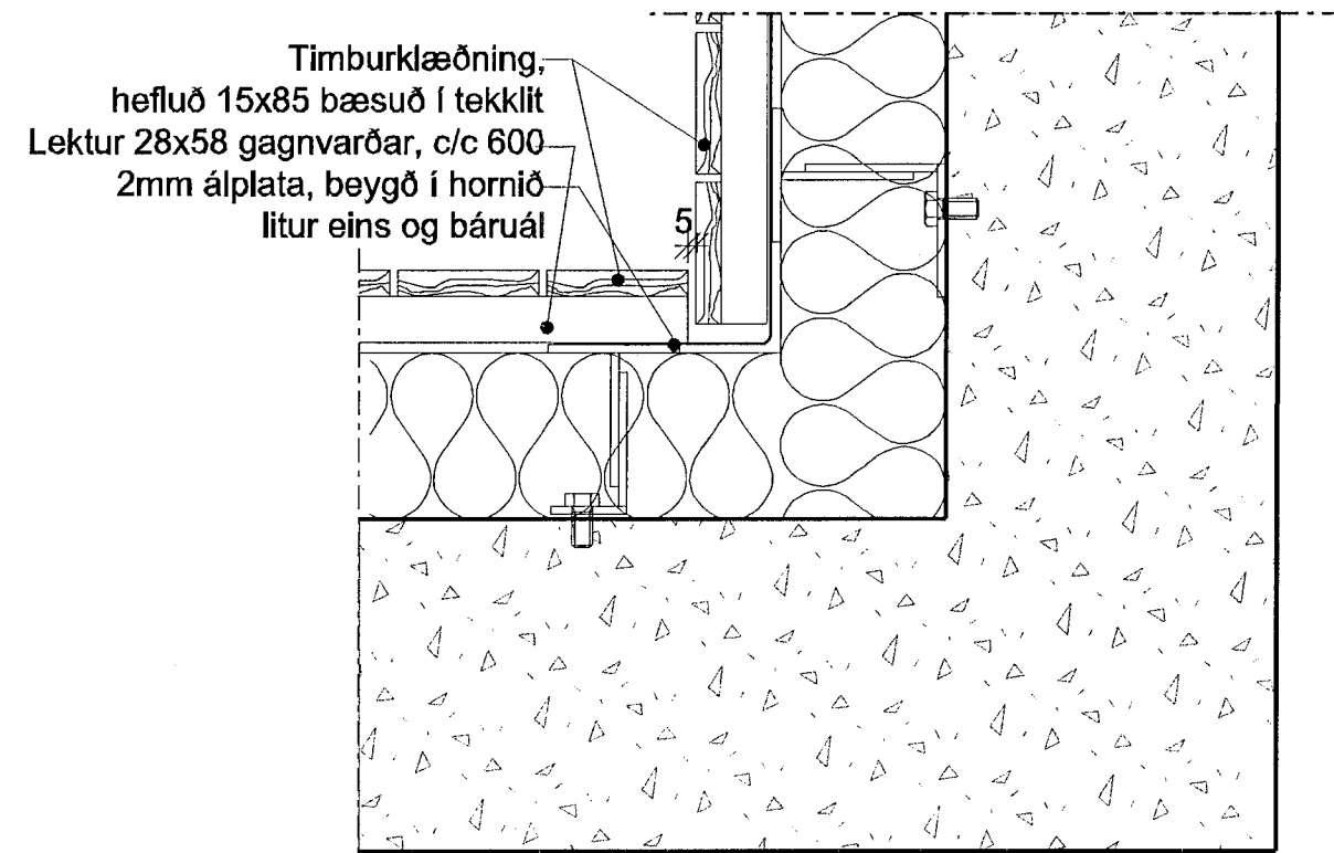
7 DEILI 1:5 INNHORN VIÐUR/VIÐUR
