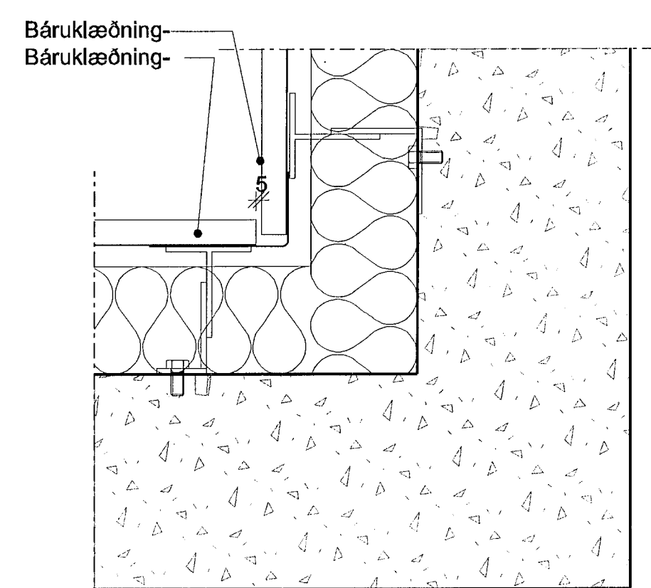
10 DEILI 1:5 INNHORN, BÁRA/BÁRA
