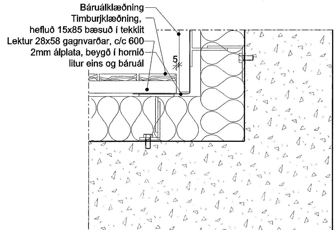
3 DEILI 1:5 INNHORN, BÁRA/VIÐUR
