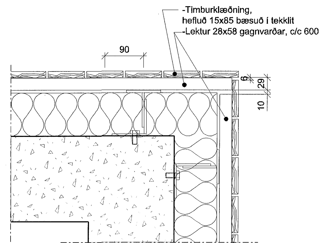
8 DEILI 1:5 ÚTHORN, VIÐUR/VIÐUR
