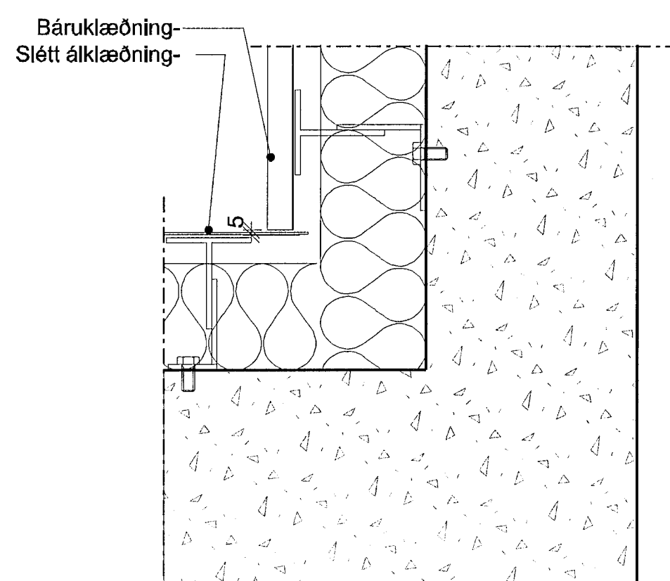
5 DEILI 1:5 INNHORN SLÉTT/BÁRA
