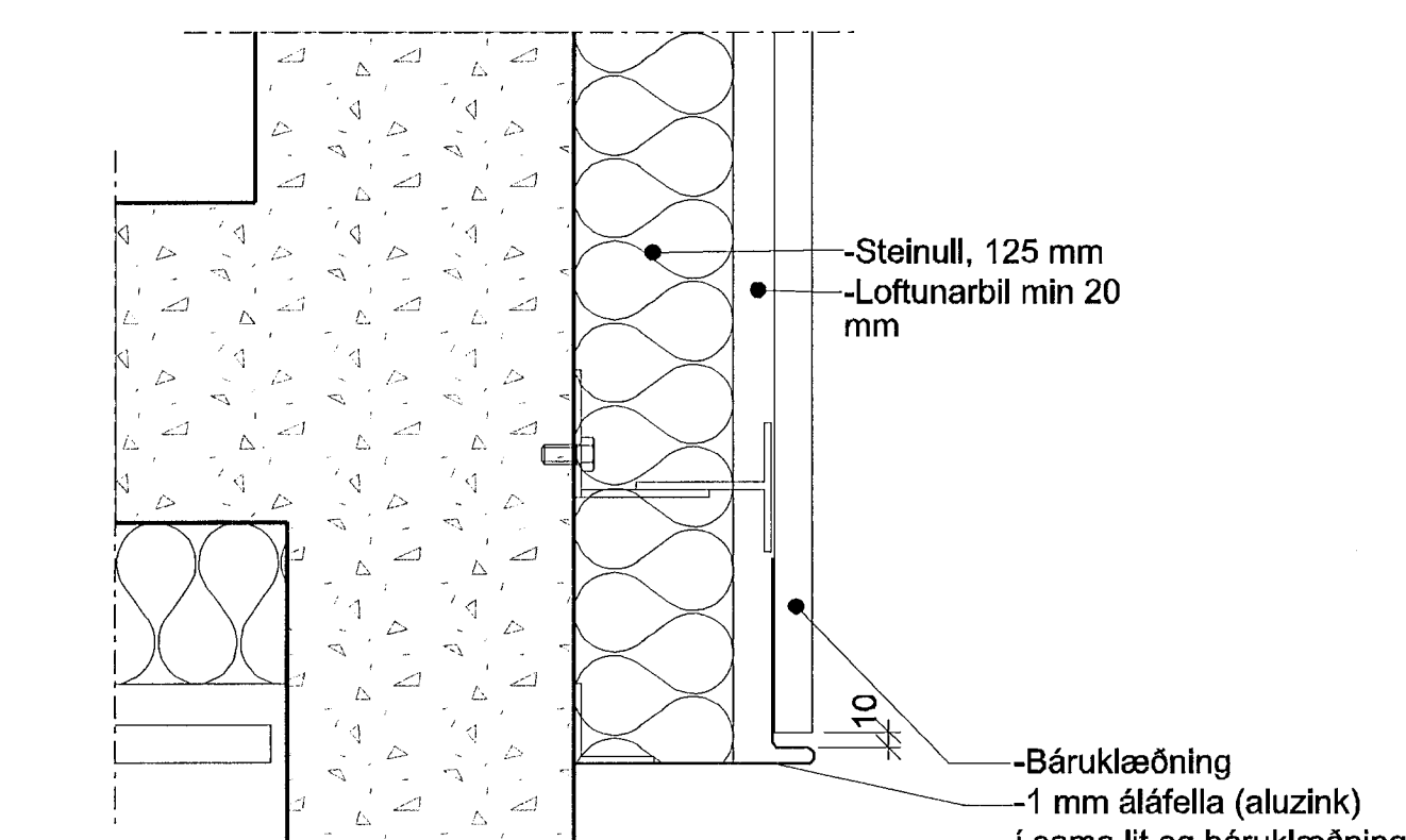
11 DEILI 1:5 BÁRA, LOKUN Á EINANGRUN
