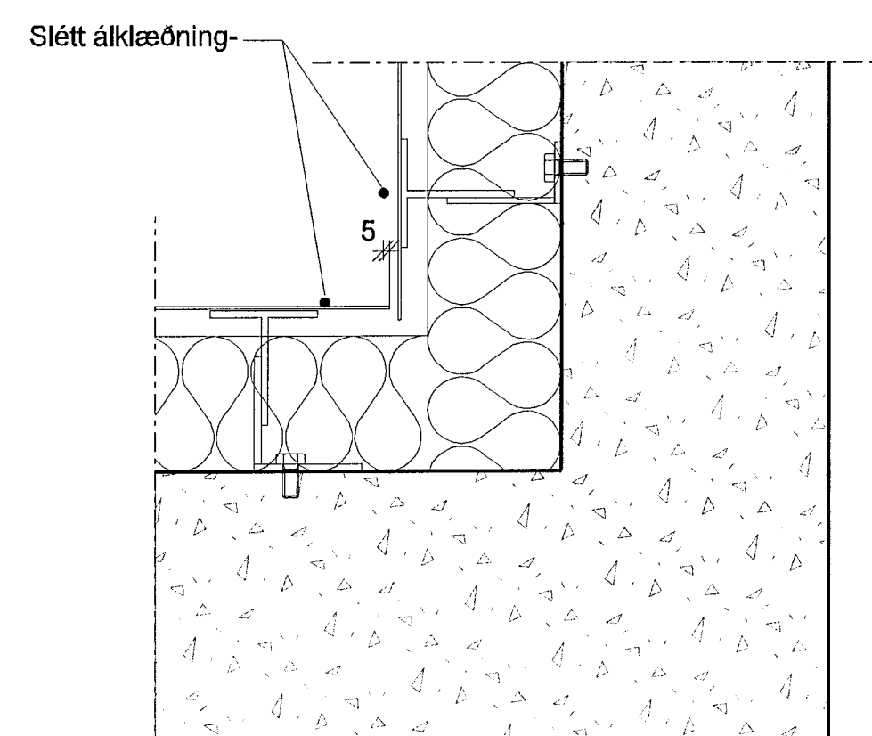
9 DEILI 1:5 INNHORN, SLÉTT/SLÉTT
