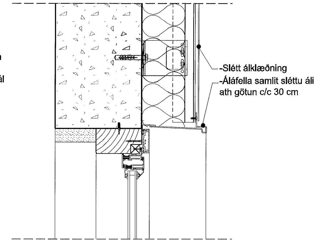
2 DEILI 1:5 Efri brún glugga m. slétttri álklaðningu (Lóðrétt deili)
