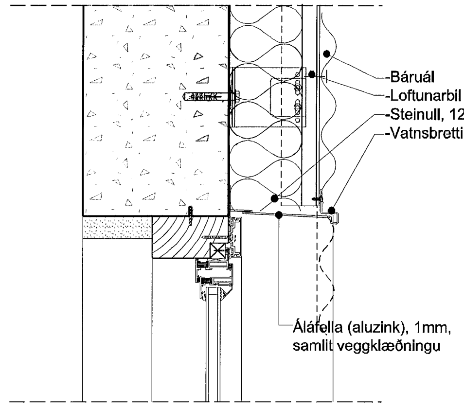
1 DEILI 1:5 Efri brún glugga m. álbáruklæðningu (Lóðrétt deili)
