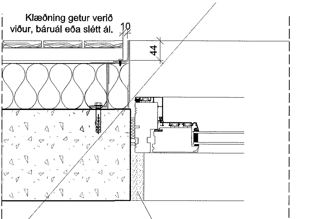
12 DEILI 1:5 Hliðarstykki hurða, eftirá ísettar (Lárétt deili)
