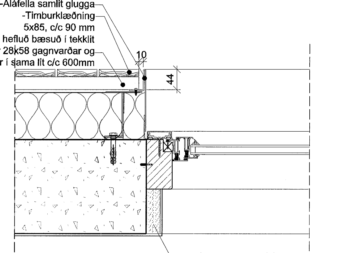
11 DEILI 1:5 Hliðarstykki glugga viðarklaðning (Lárétt deili)
