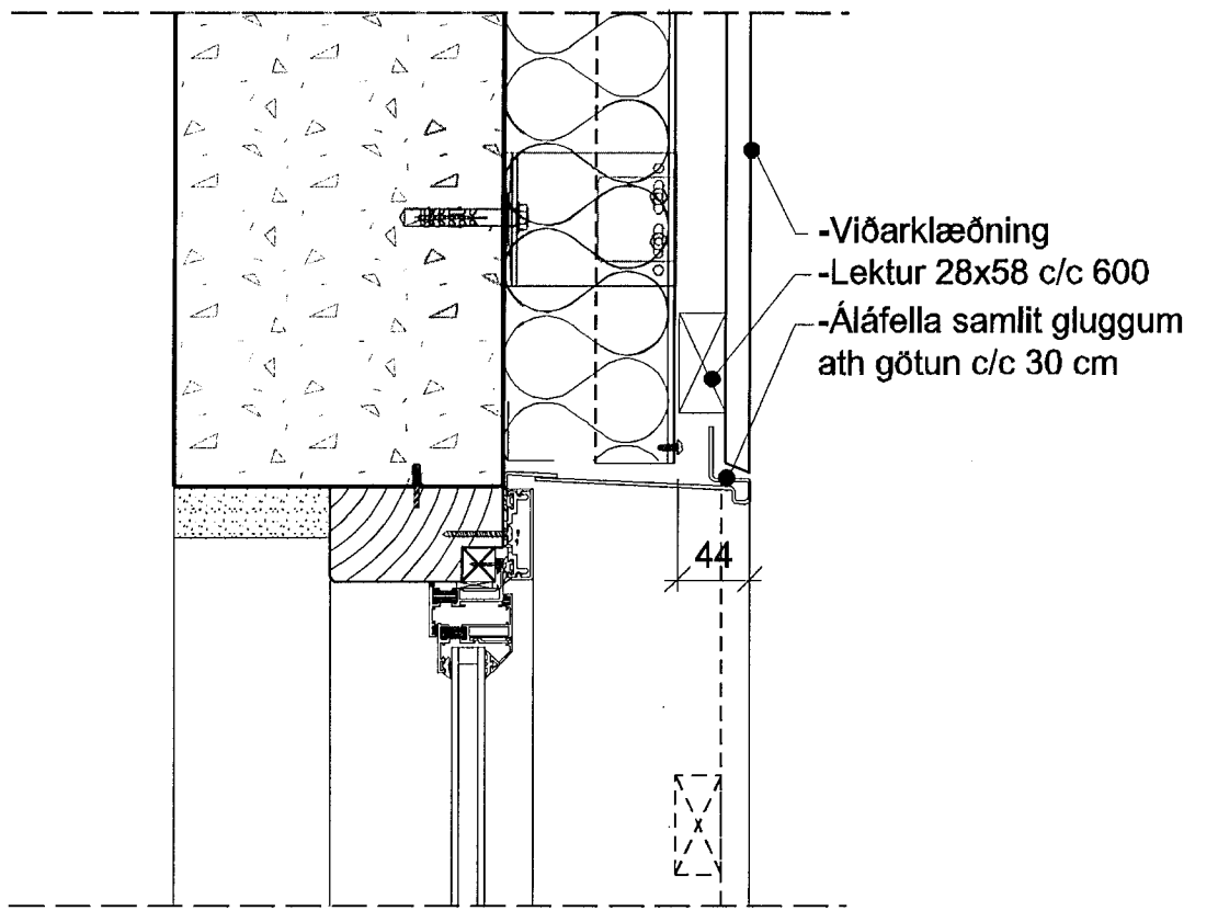
3 DEILI 1:5 Efri brún glugga, viðarklaðning
