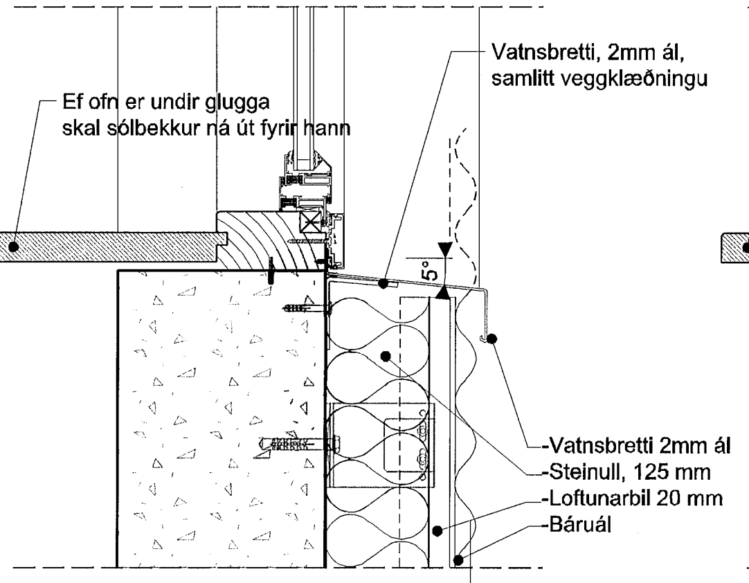
5 DEILI 1:5 Neðri brún glugga m. bárúáli (Lóðrétt deili)
