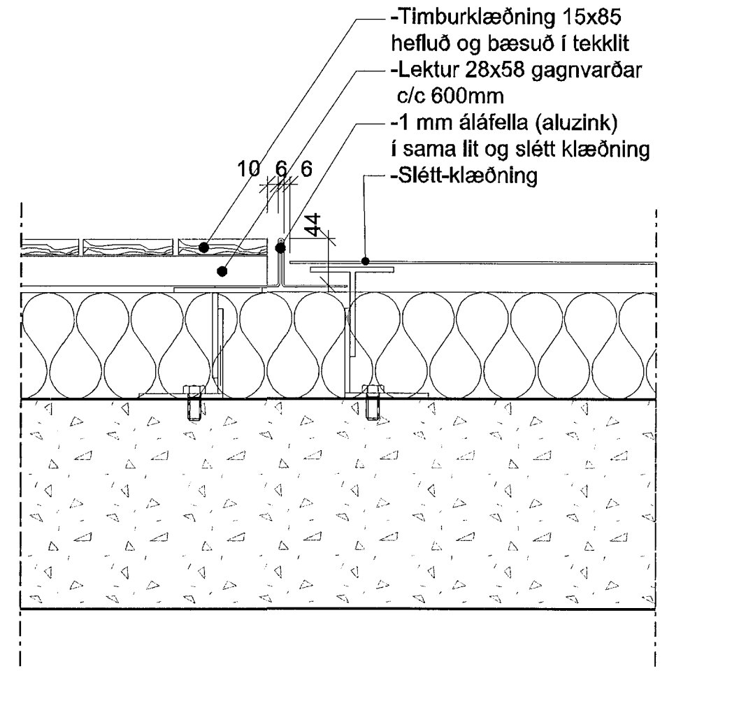
8 DEILI 1:5 Viður / Slétt (Lárétt)
