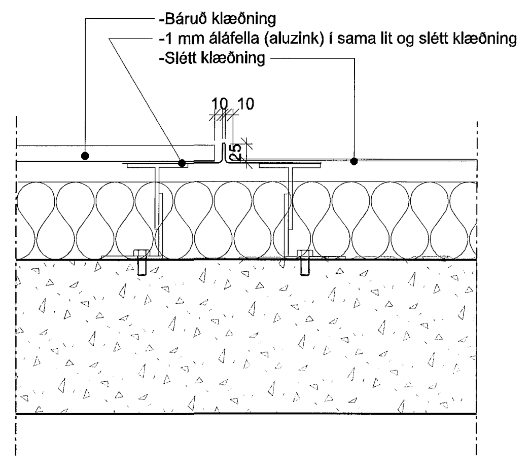
4 DEILI 1:5 Bárúál/Slétt (Lárétt)
