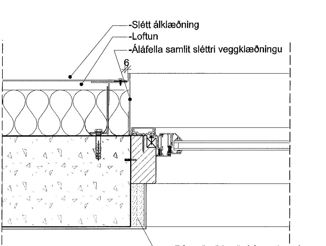
9 DEILI 1:5 Hliðarstykki glugga, slétttri álklaðning (Lárétt deili)
