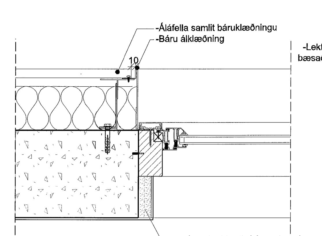
10 DEILI 1:5 Hliðarstykki glugga, bárúálklæðning (Lárétt deili)
