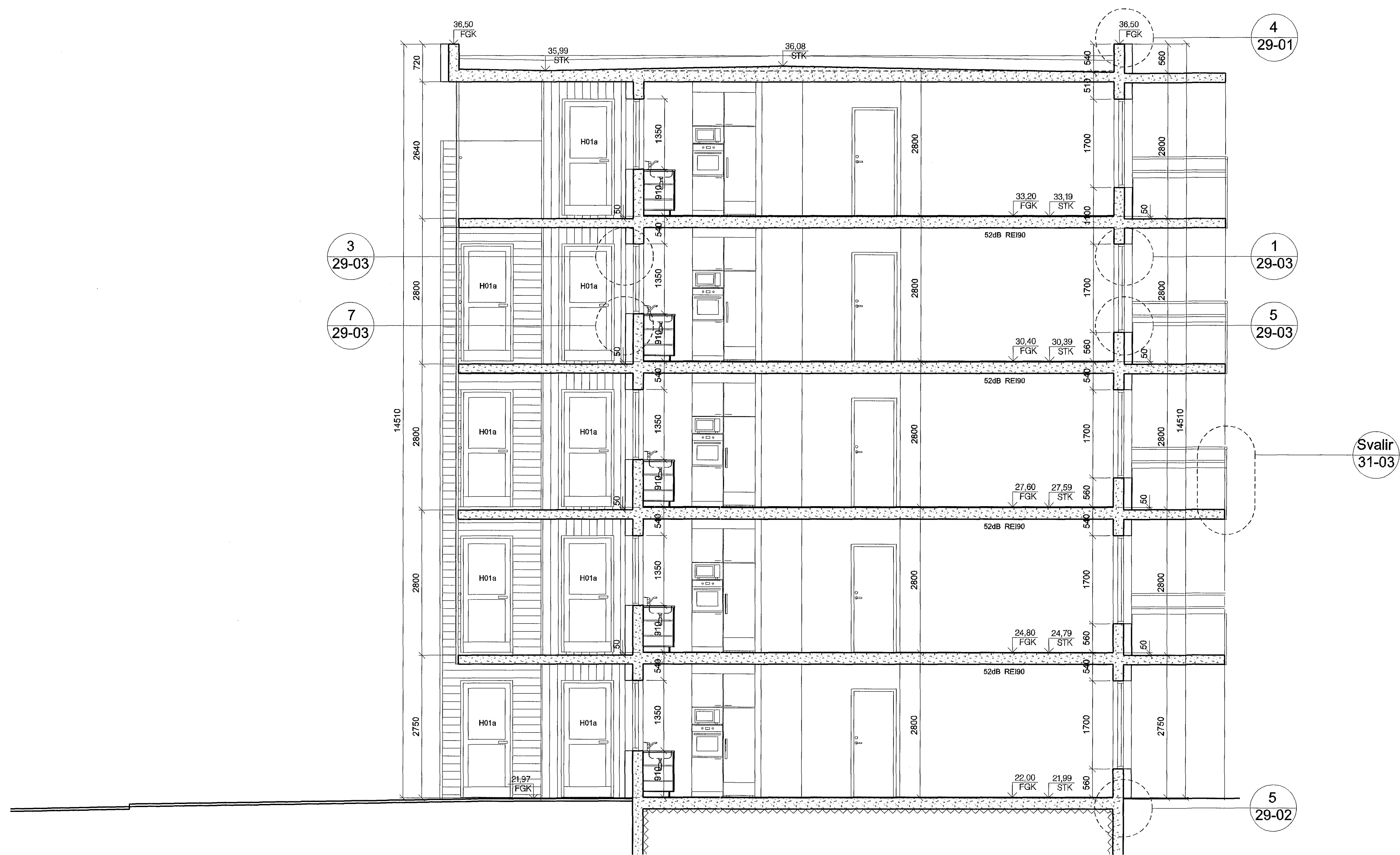
G-G 20-02 20-04 20-06 20-08 20-10 20-12 20-14 SNEIÐING 1:50
