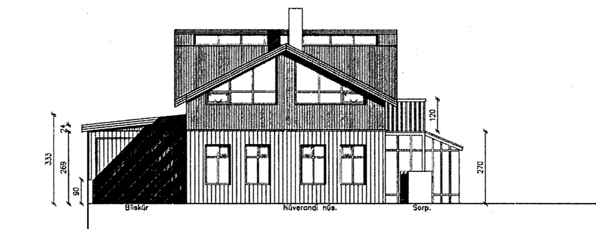
Útlit SUDUR. 1:100
