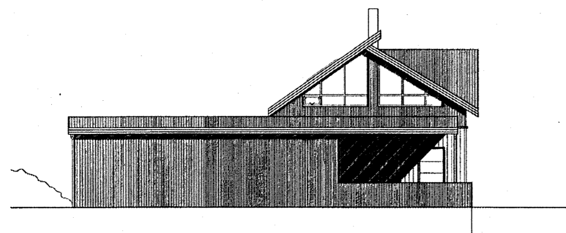
Útlit VESTUR. 1:100
