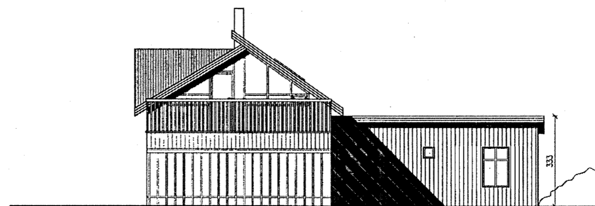
Útlit AUSTUR. 1:100
