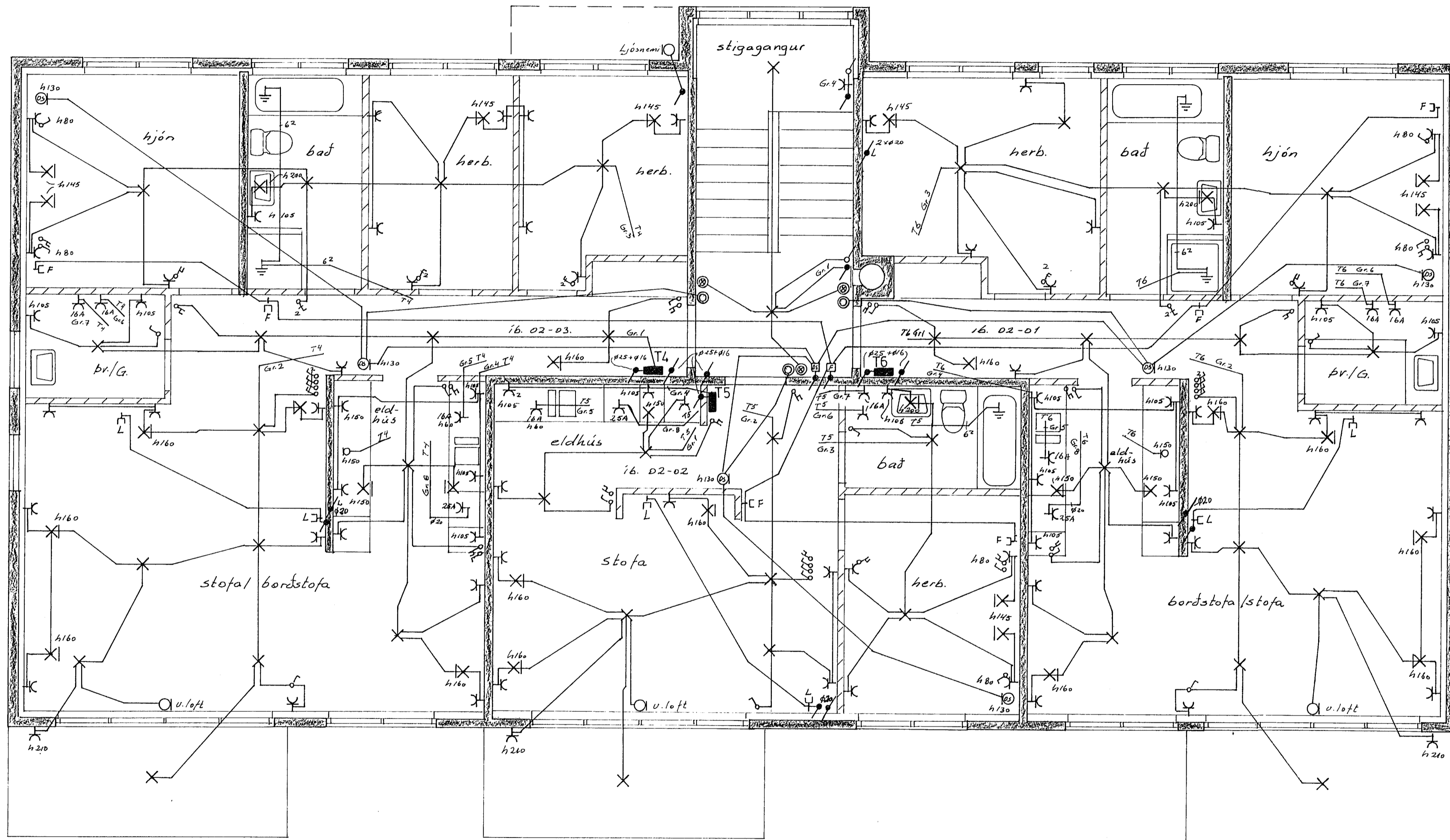
2. HÆÐ M 1:50
