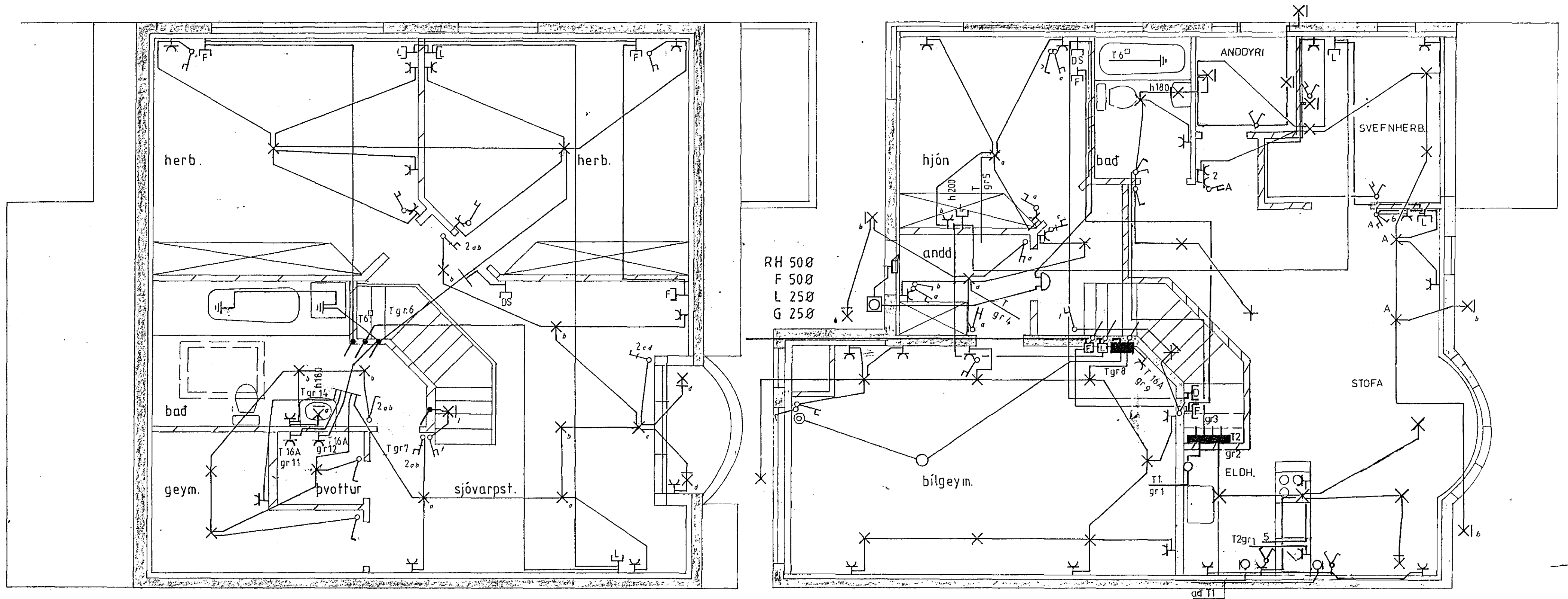
Grunnmynd efri hæð mkv. 1:50
