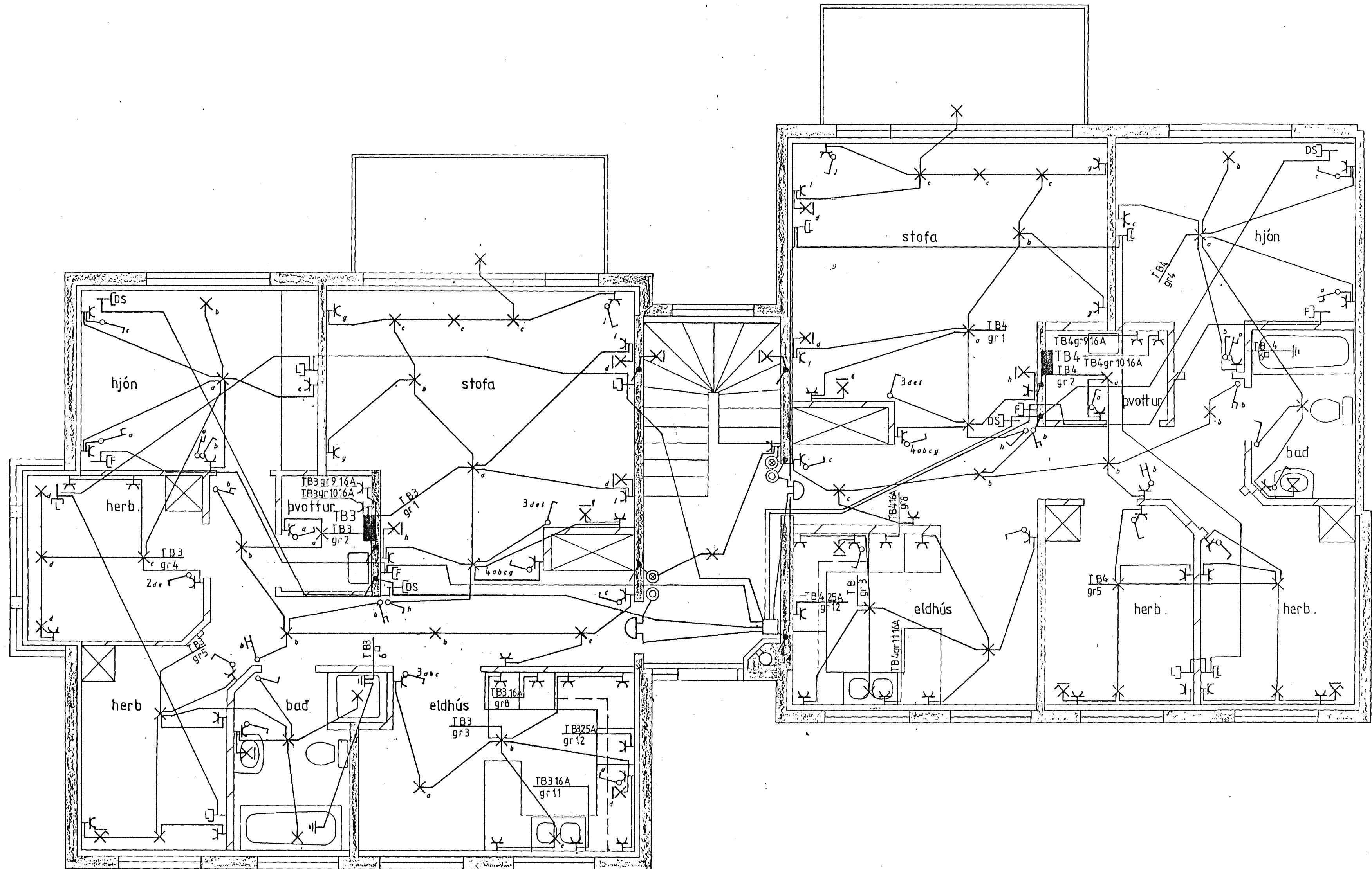
Grunnmynd 2 hæð mkv.1:50
