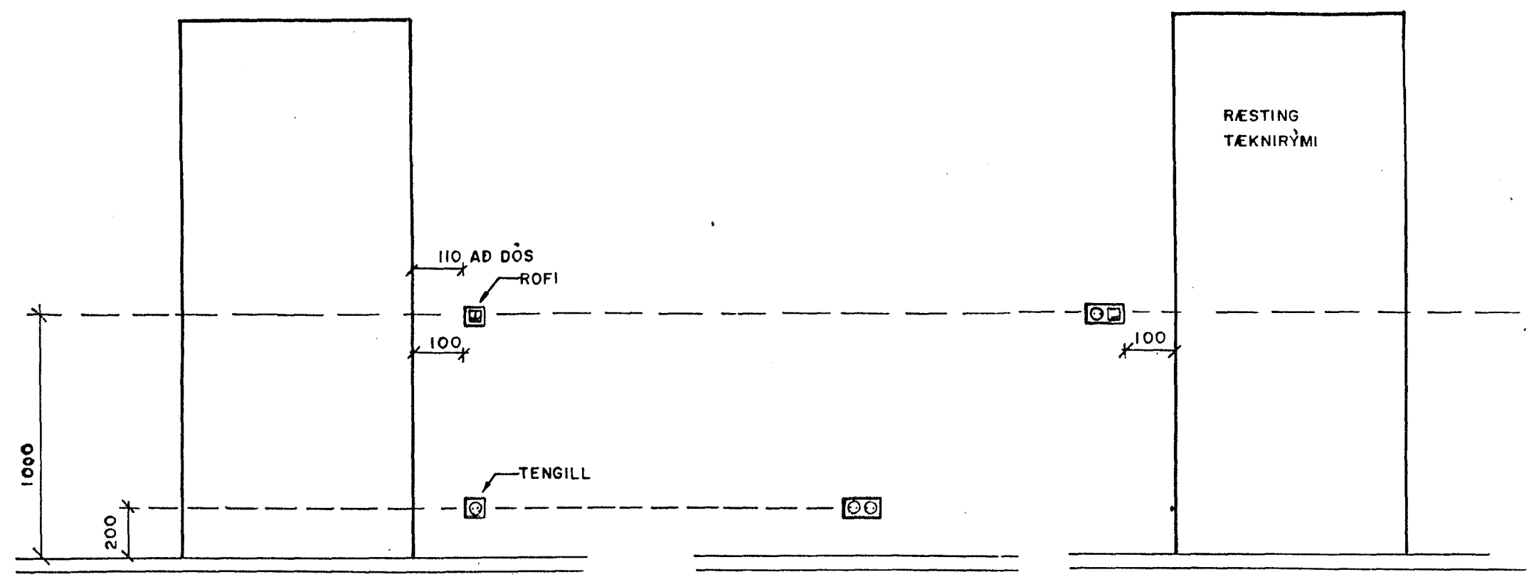
M 1:20 DEMIGERÐ MÁLSETNING Á ROFUM OG TENGLUM
