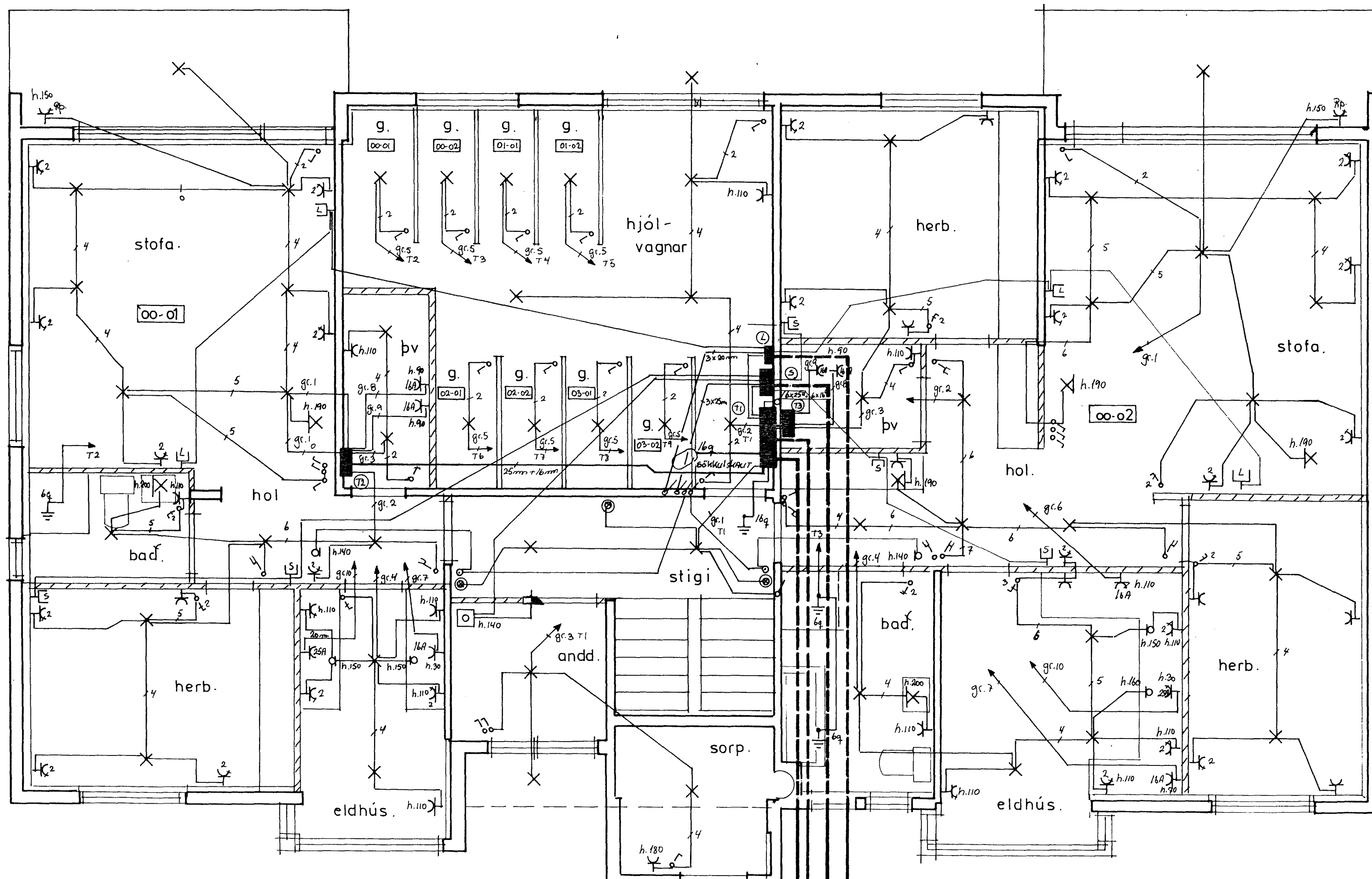
GRUNNMYND JARÐHÆÐ MÁL 1:50
