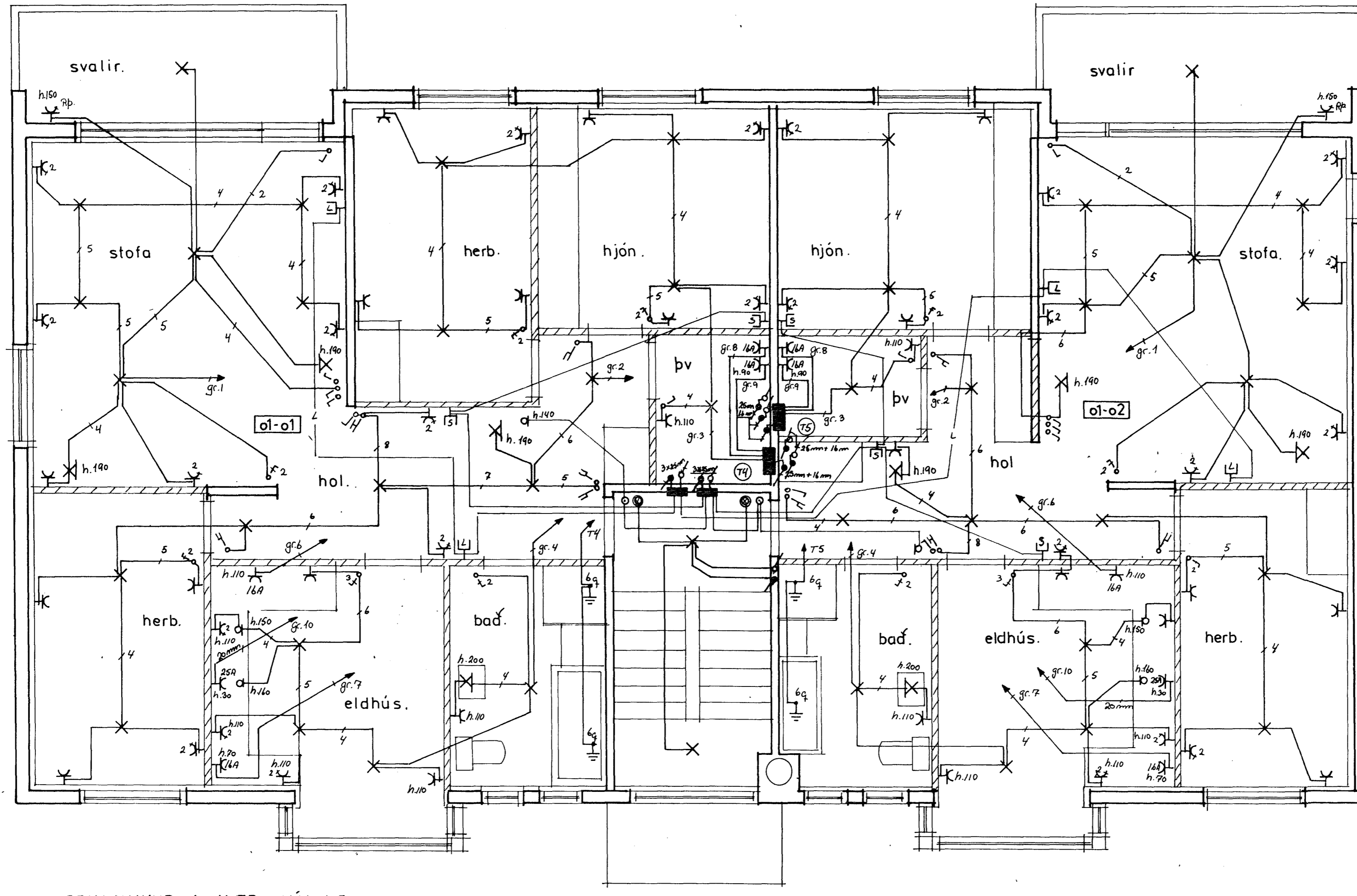
GRUNNMYND 1. HÆÐ MÁL 1:50
