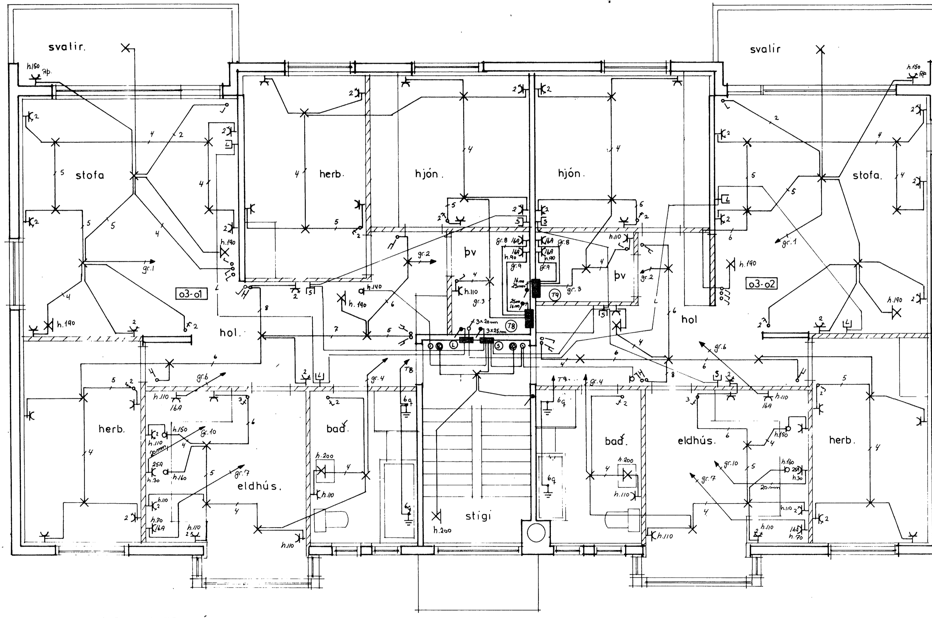
GRUNNMYND 3. HÆÐ MÁL 1:50
