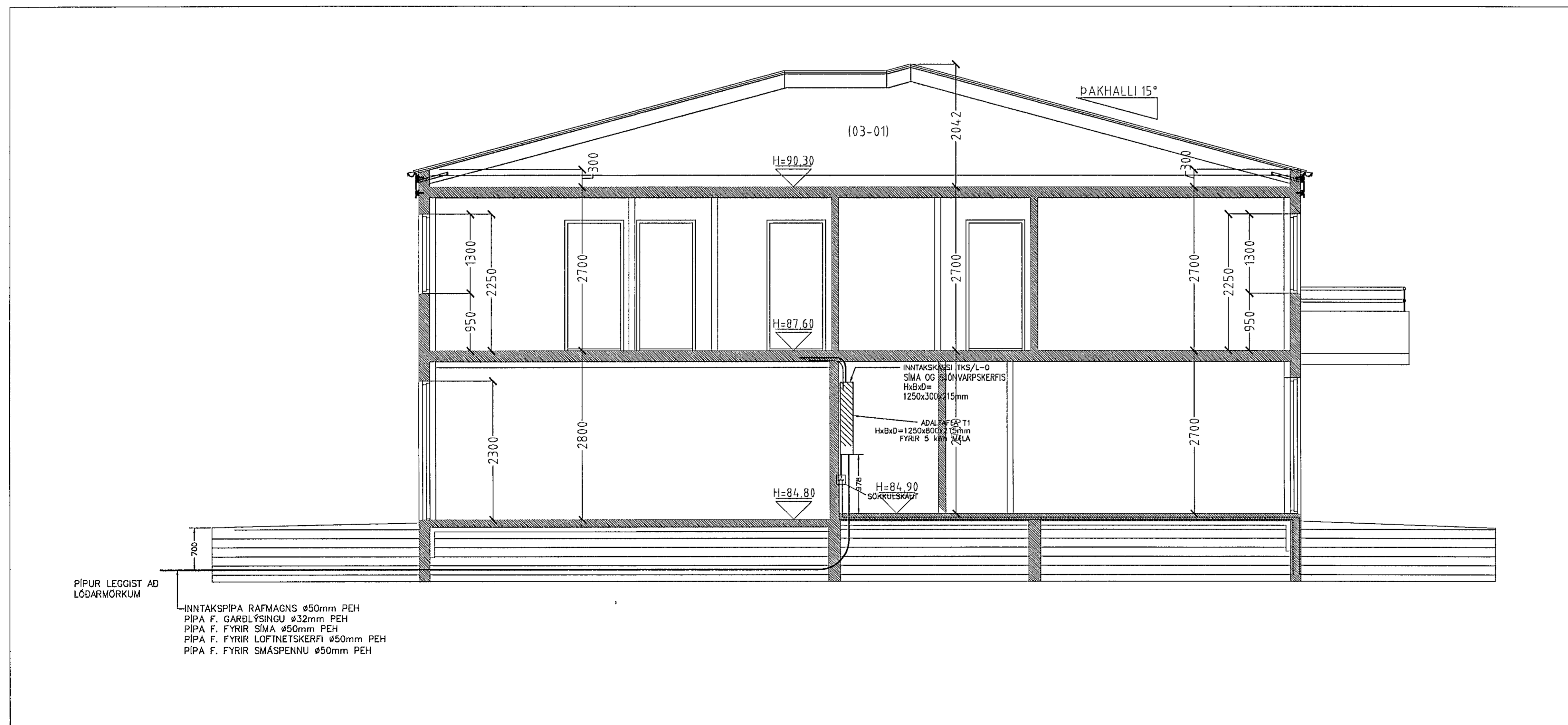
A SNID Í INNTAKSHERBERGI 2-3 MKV. 1:50
