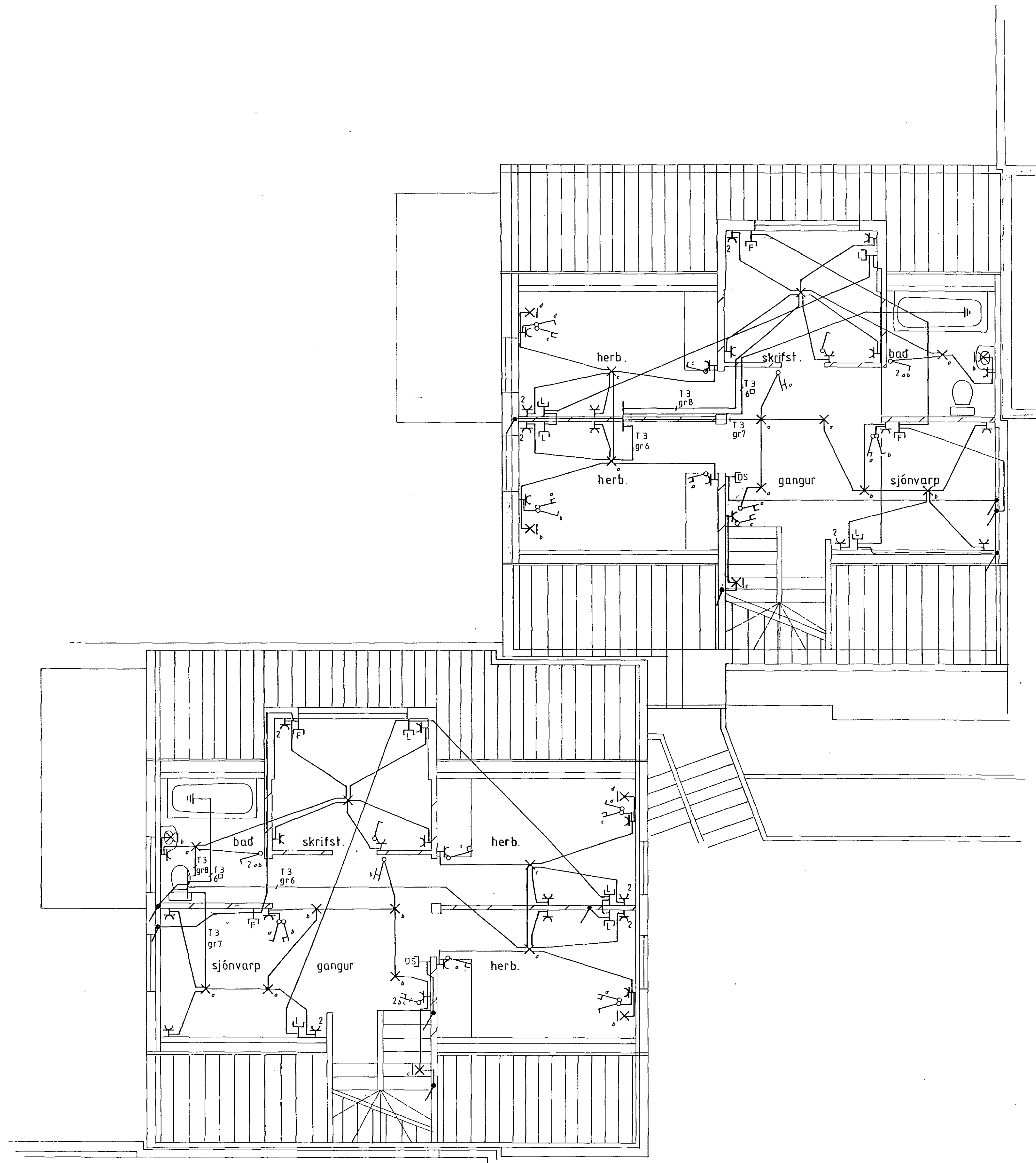
Grunnmynd ris mkv 1:50
