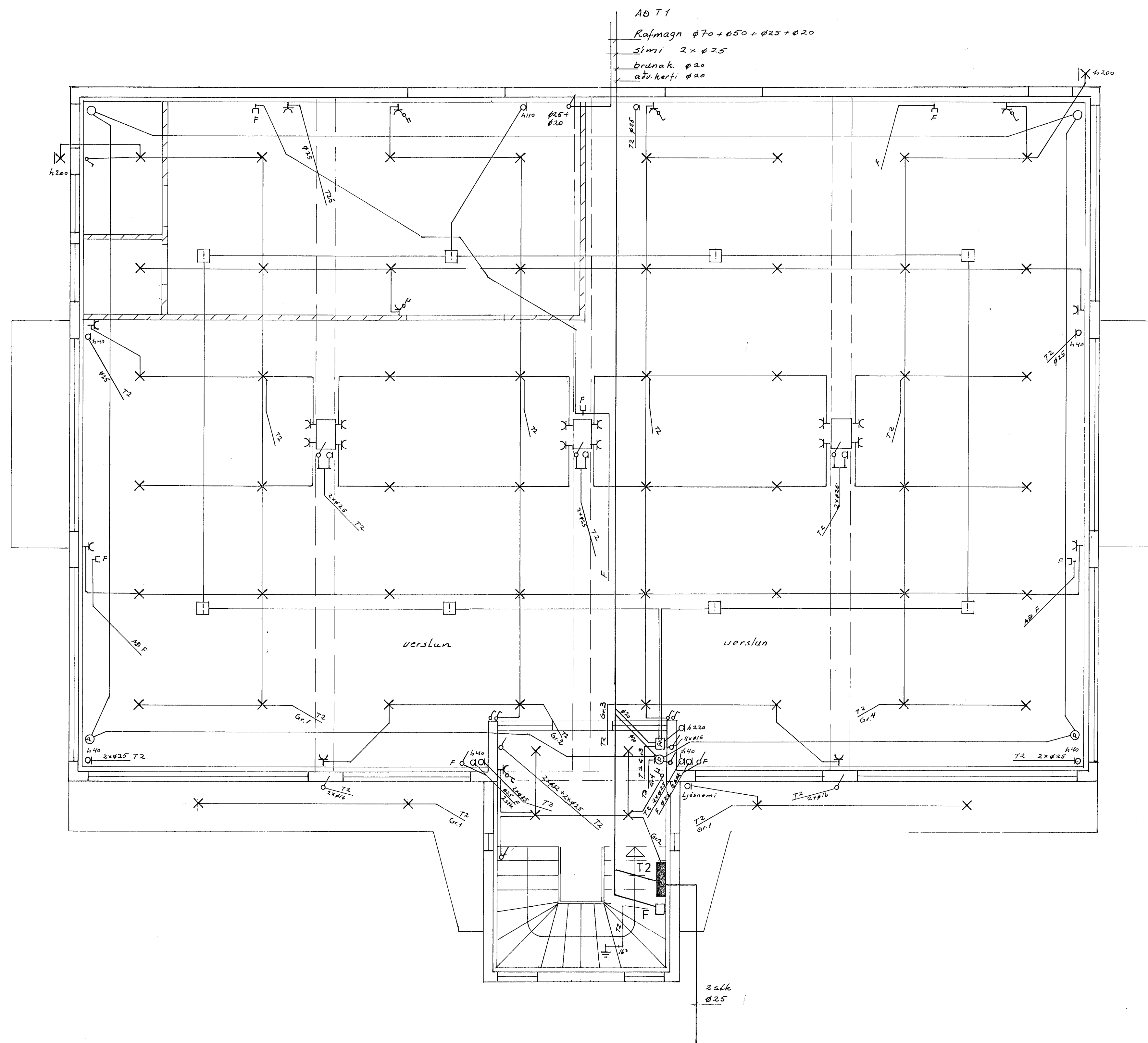
1. HÆÐ M 1:50
