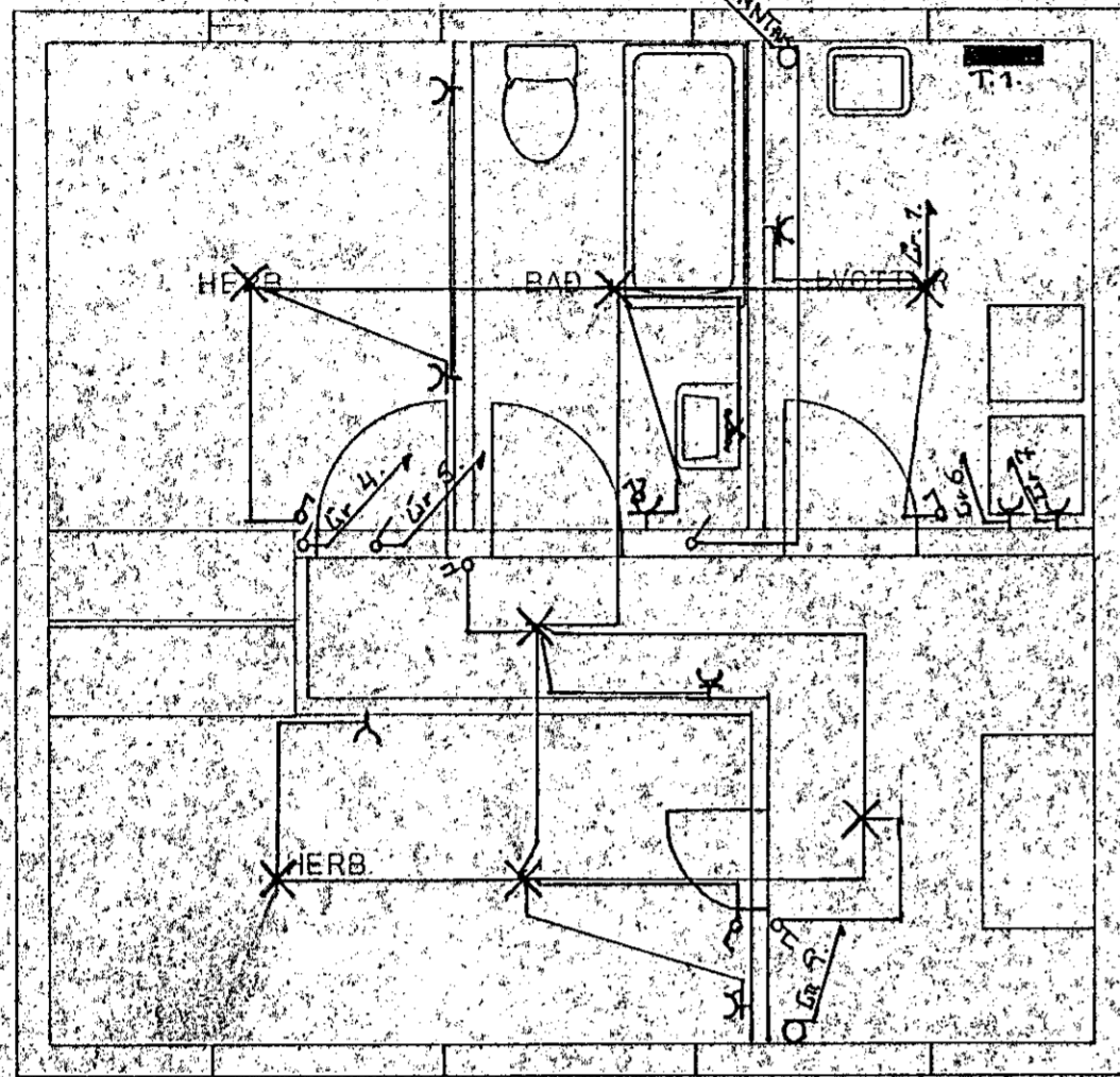
GRUNNMYND KJALLARA 1:50
