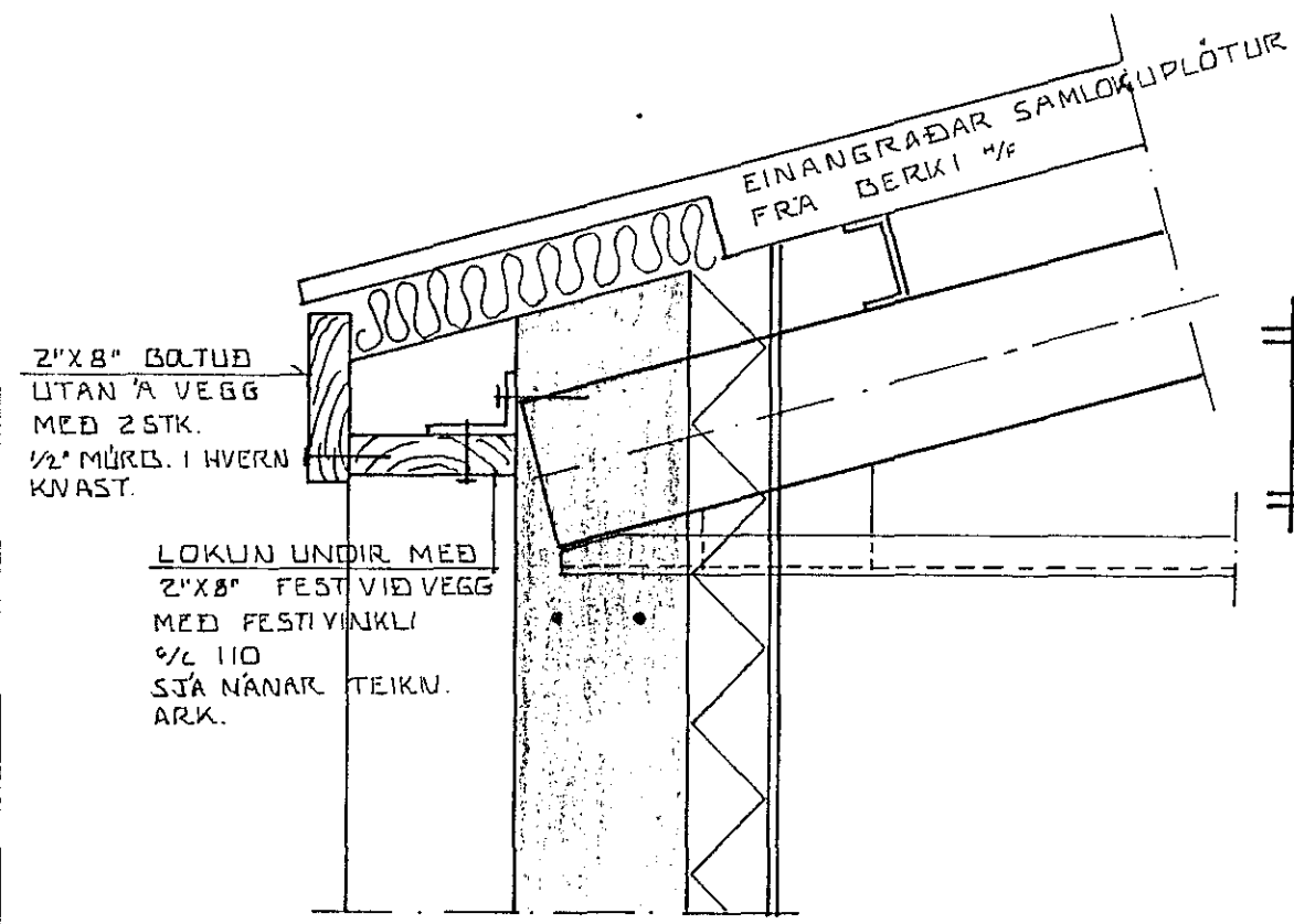
SNID VID ÞAKBRÚN 1:10
