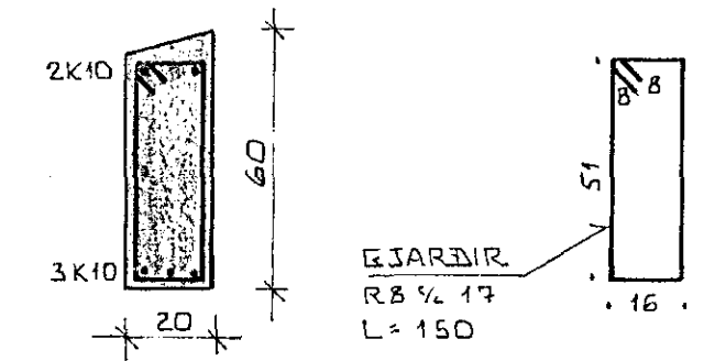
BITI YFIR HURD SNID A-A ~ 1:20
