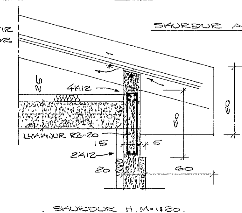
SKURÐUR H, M=1:20
