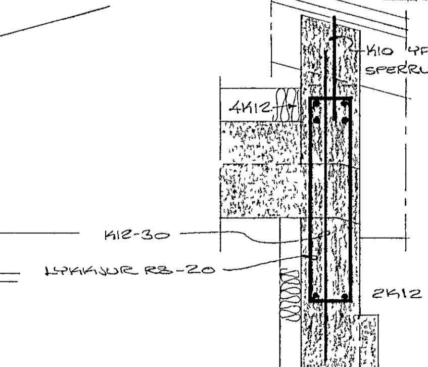
SKURÐUR H, M=1:10
