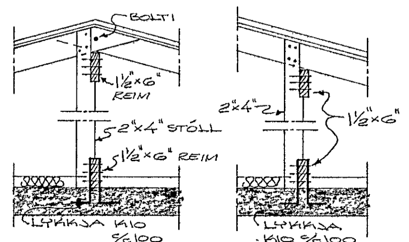
SKURDUR D, M=1:20 SKURDUR E, M=1:20
