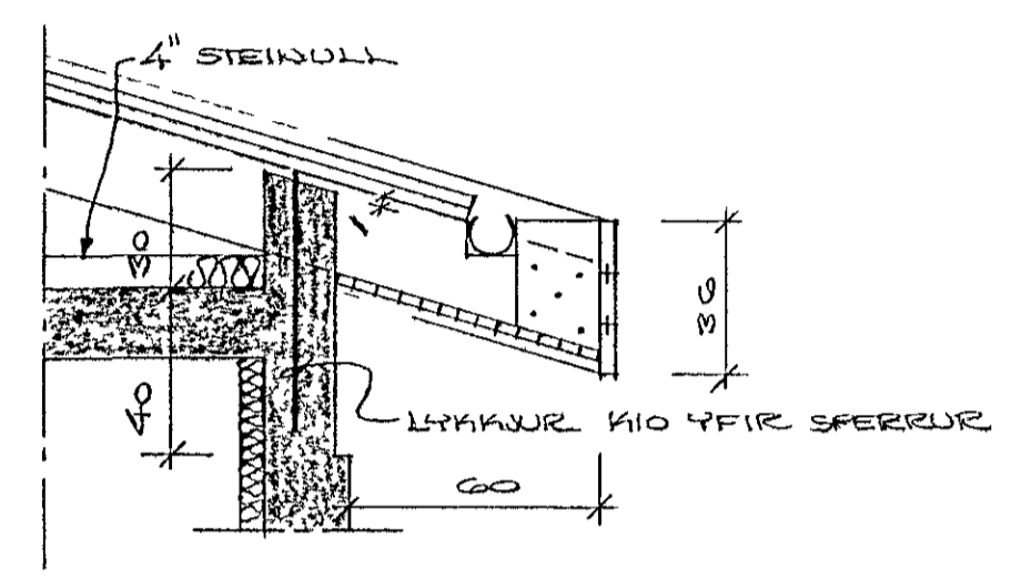
SKURDUR A, M=1:20
