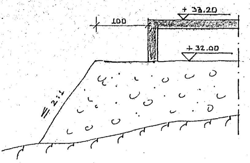
SNID A-A 1:50
