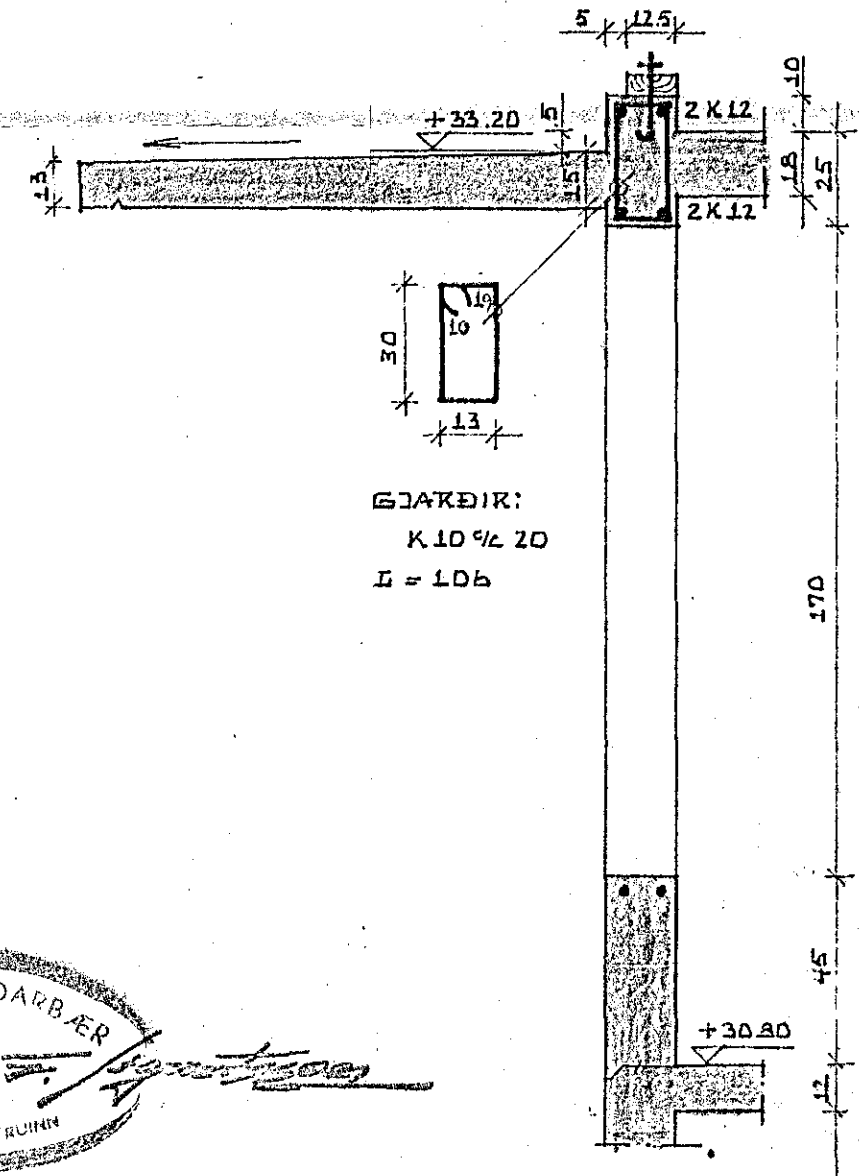
SNID A-A 1:20
