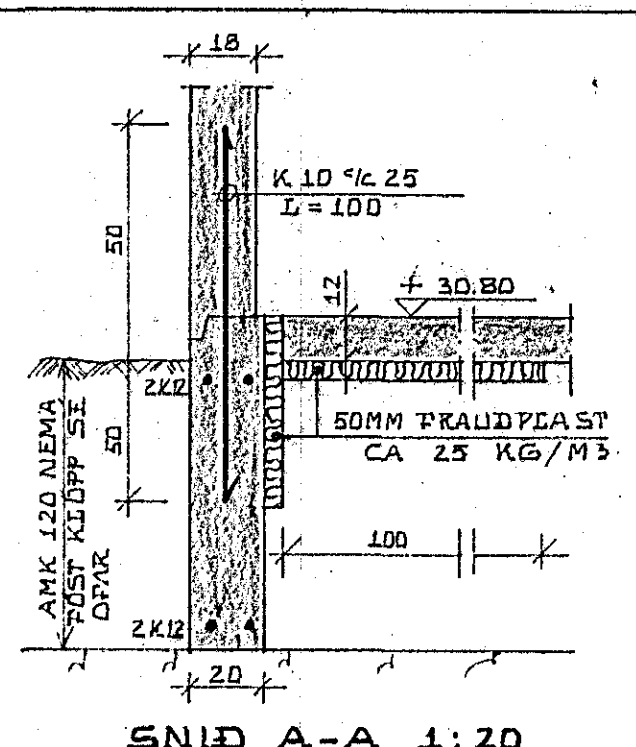
SNID A-A 1:20
