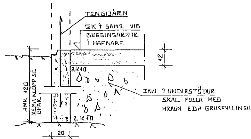
KENNISNIÐ Í UNDIRSTÖÐUR 1:20.
