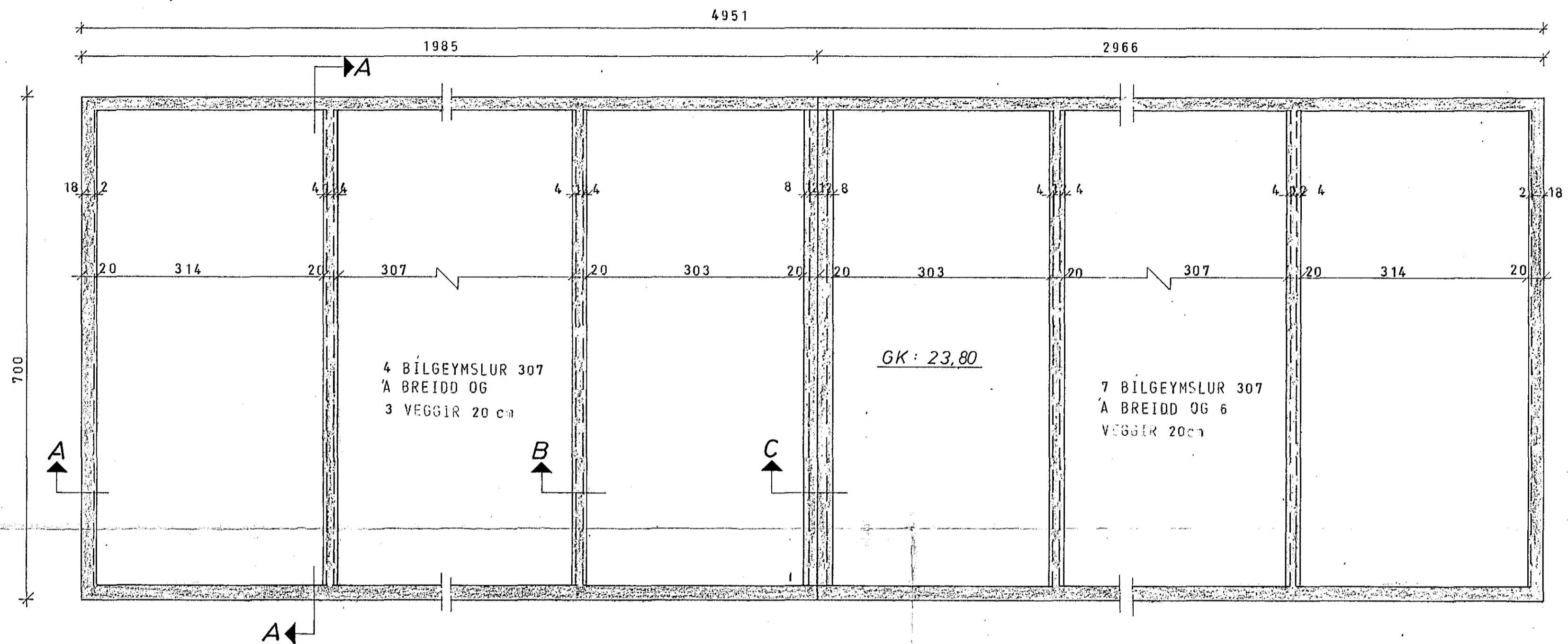
GRUNNMYND 1:50
