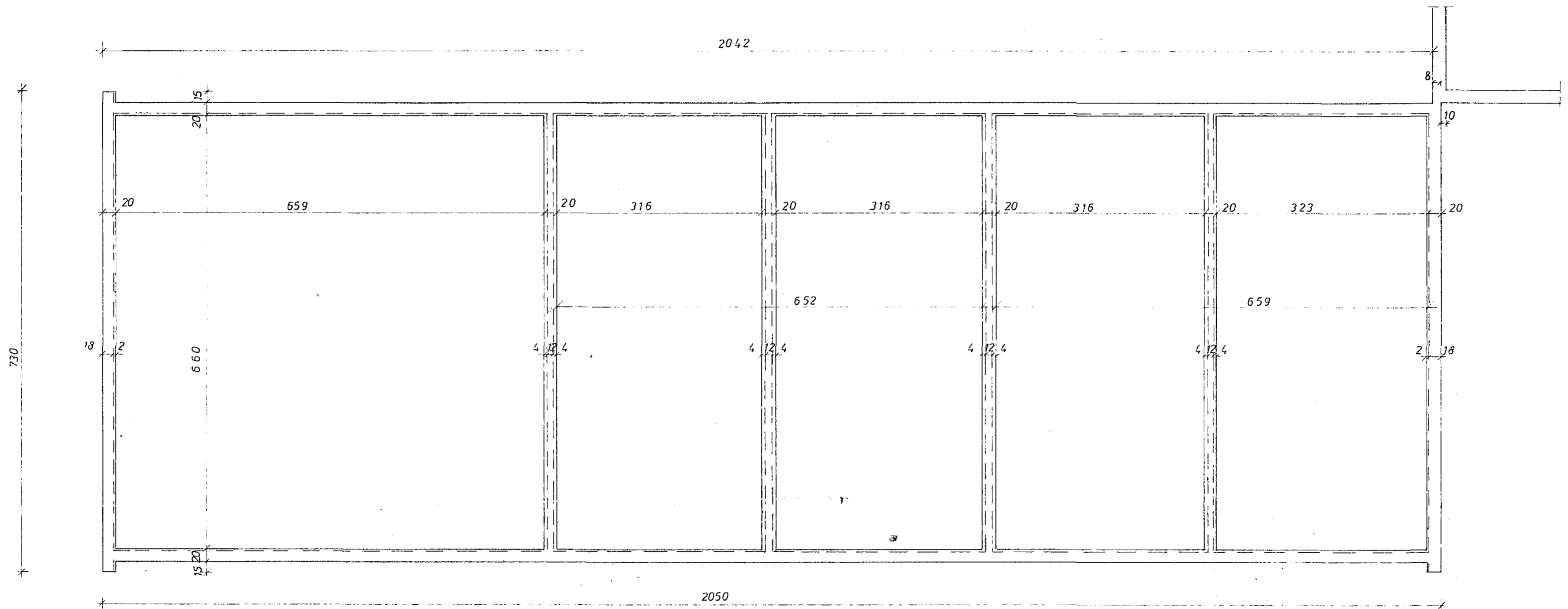
GRUNNMYND 1:50
