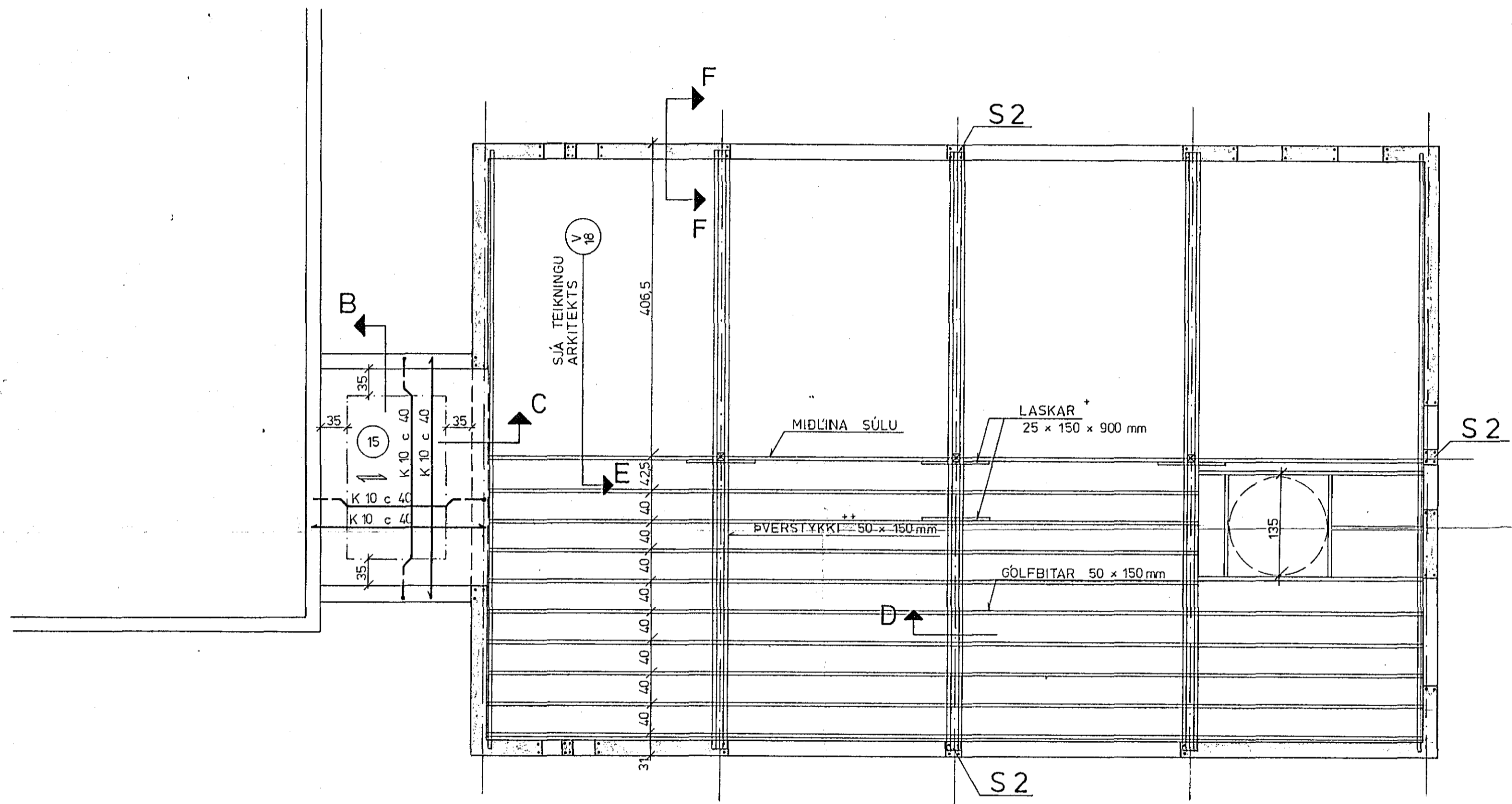
GRUNNMYND 1 : 50
