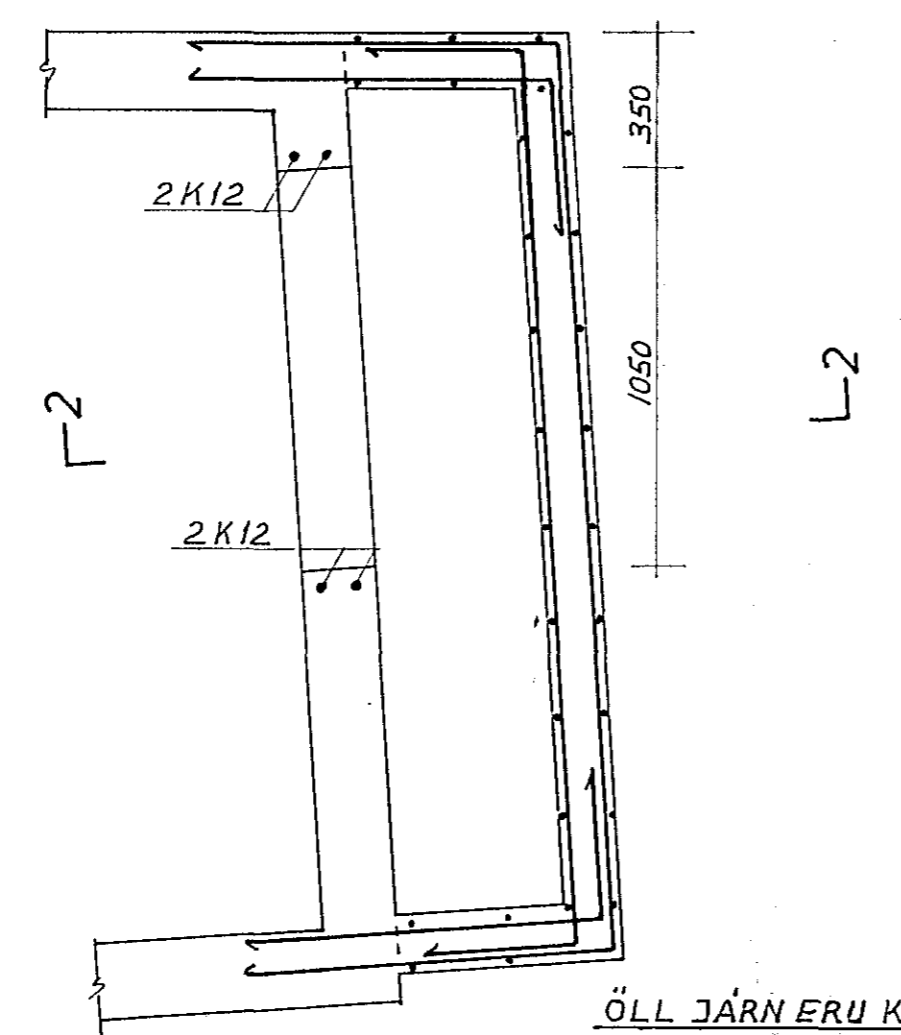
SNID 1-1 1:20
