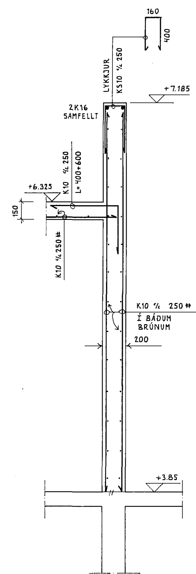
SNID A-A 1:20
