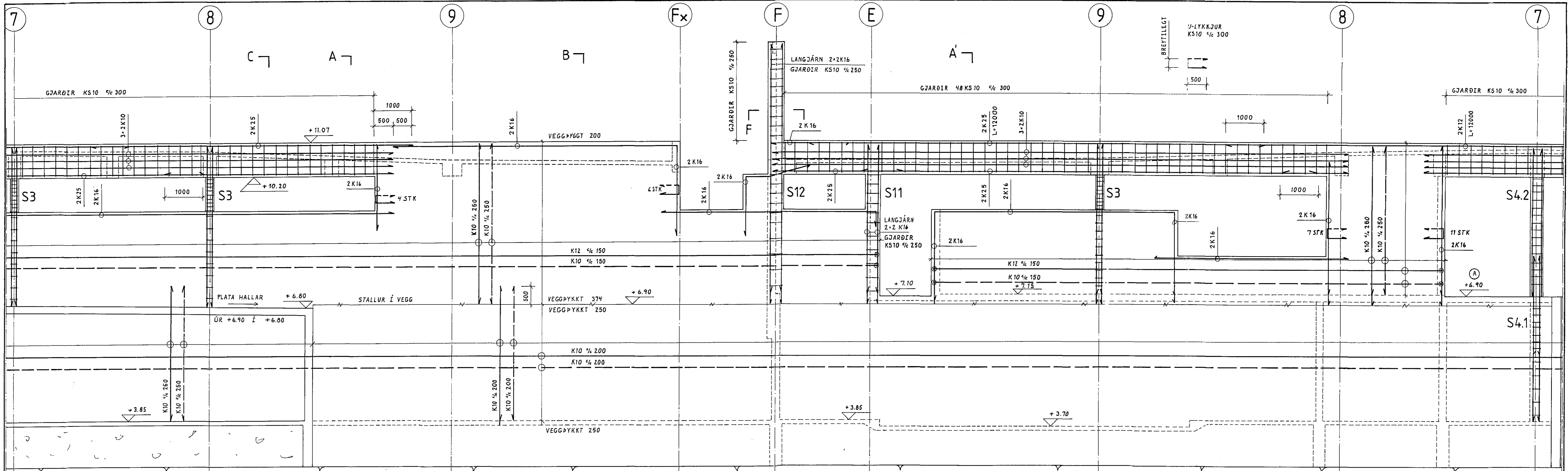
EYSTRI HLUTI ÚTVEGGJAR 1:50 ÚTFLATT
