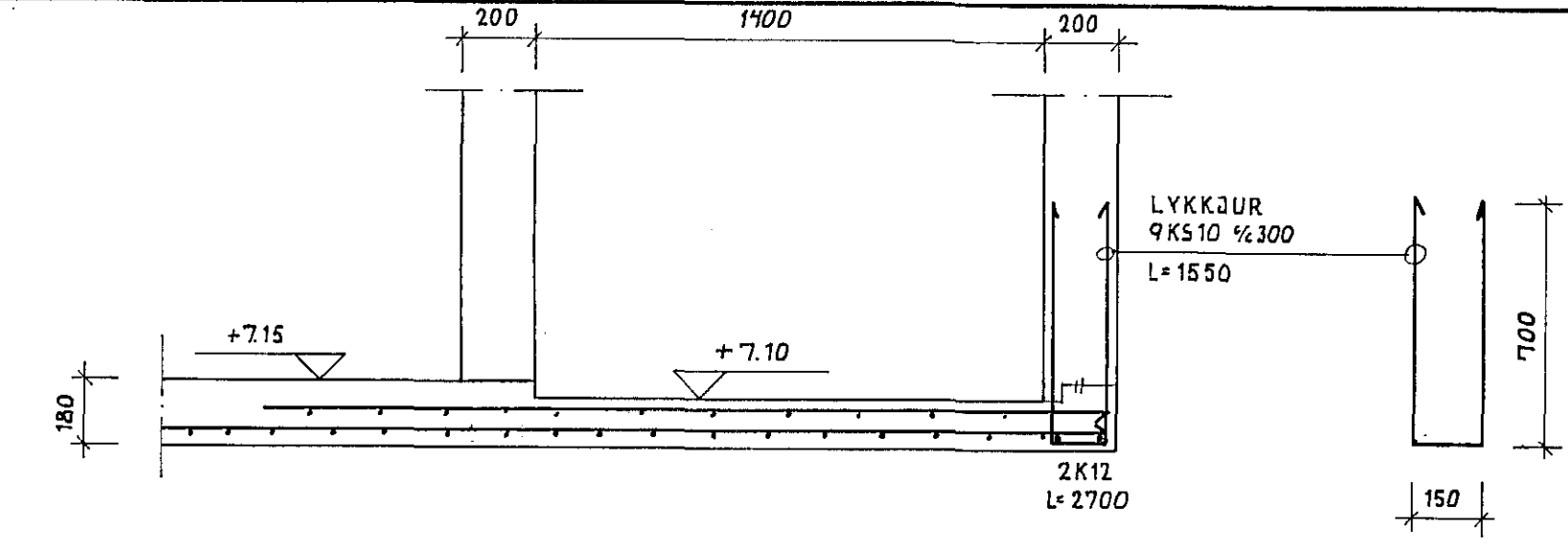
SNID A-A 1:20
