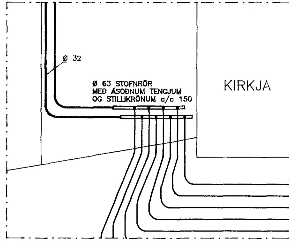
GRUNNMYND 1:50
