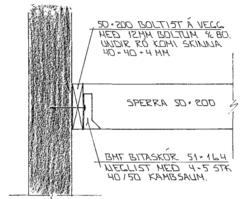
SÉRMÝND A • 1:10
