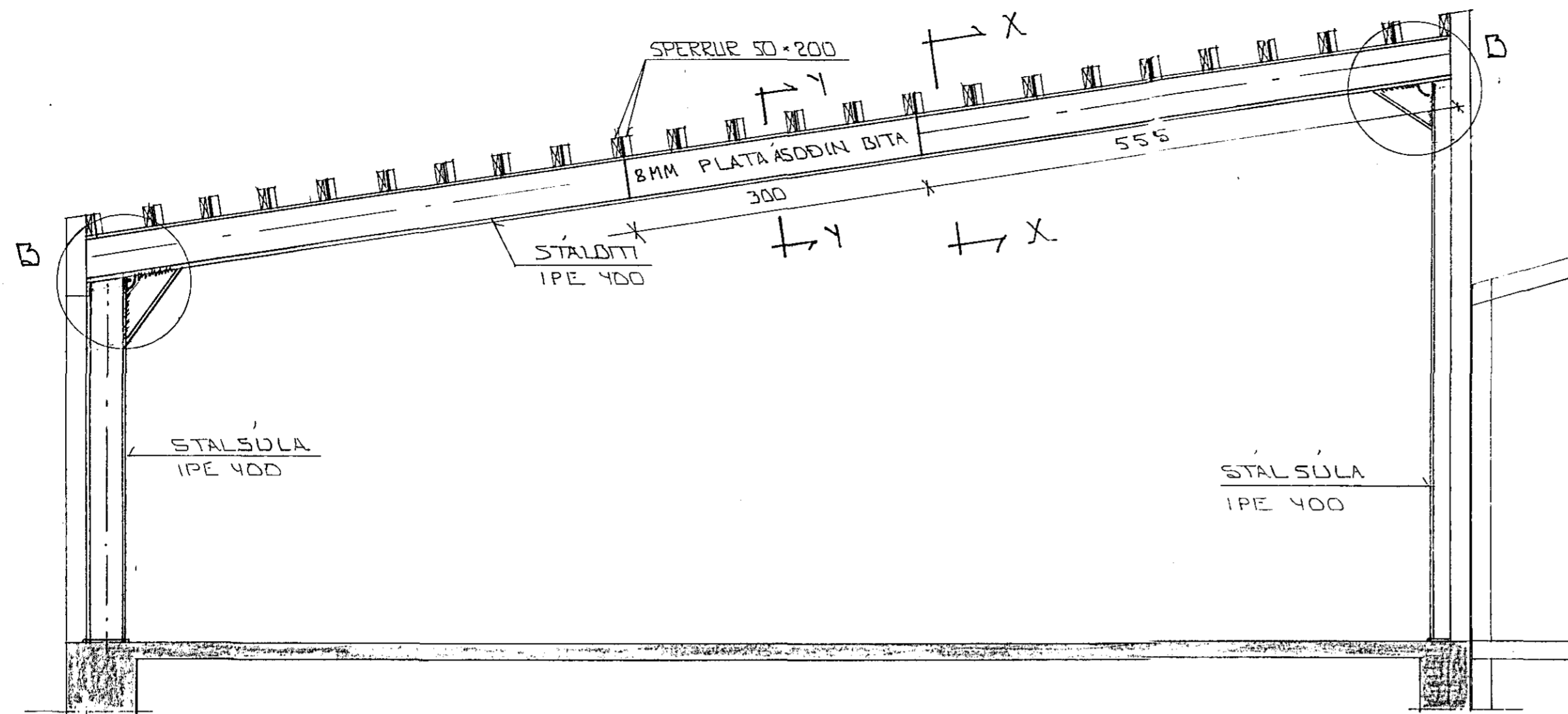
SNIÐ 3-3 • 1:50
