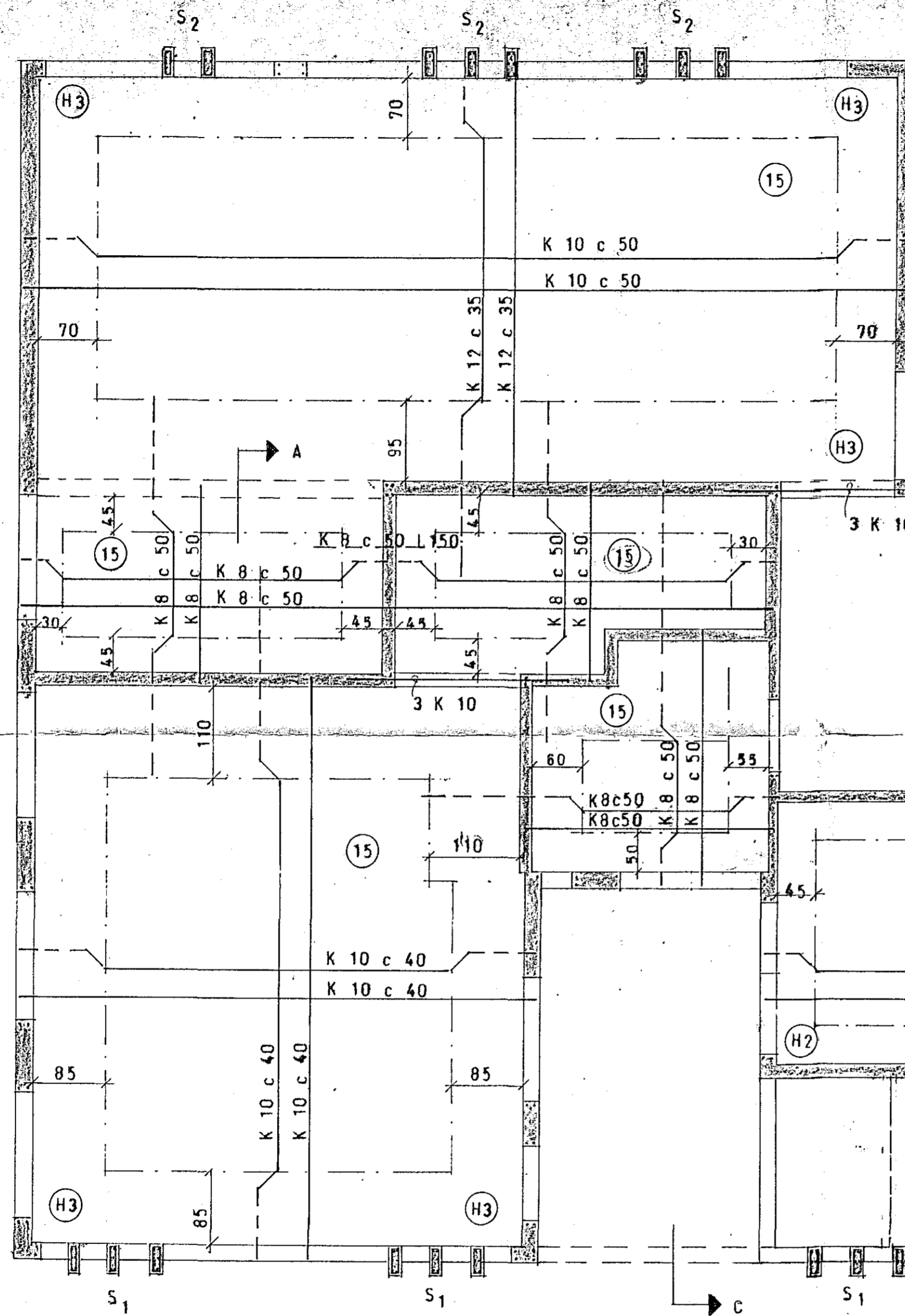
ÞRUNNMYND 1 : 50
