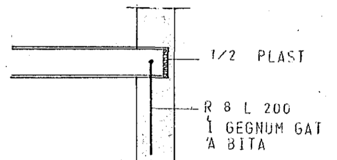
FESTING Á STÁLBITA 1:20
