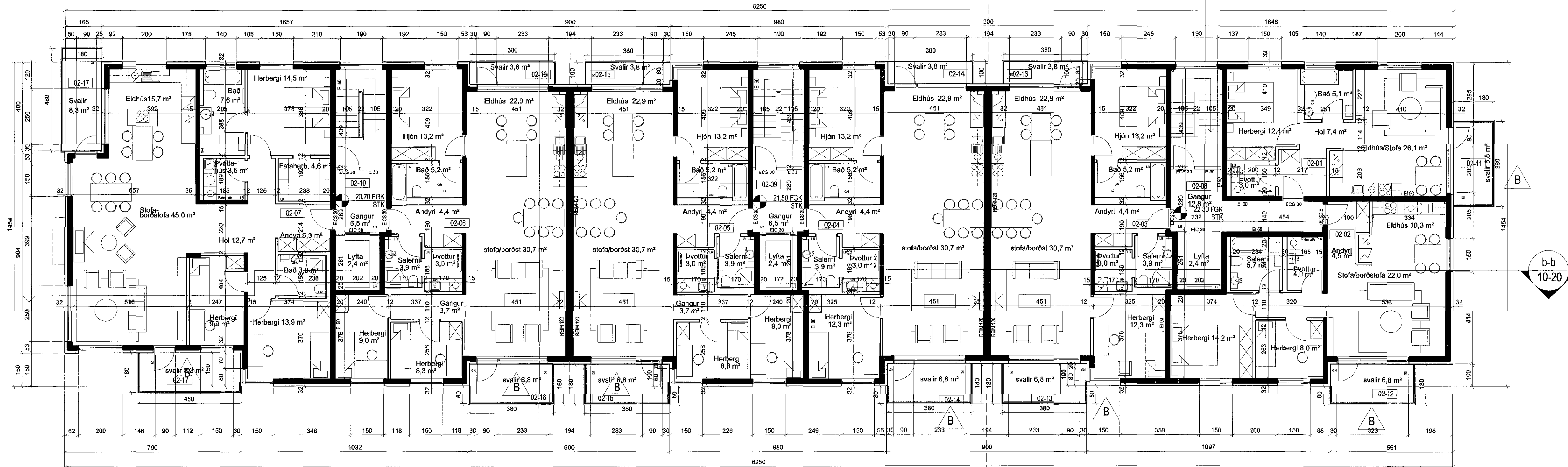
GRUNNMÝND 2. HÆÐ 1:100
