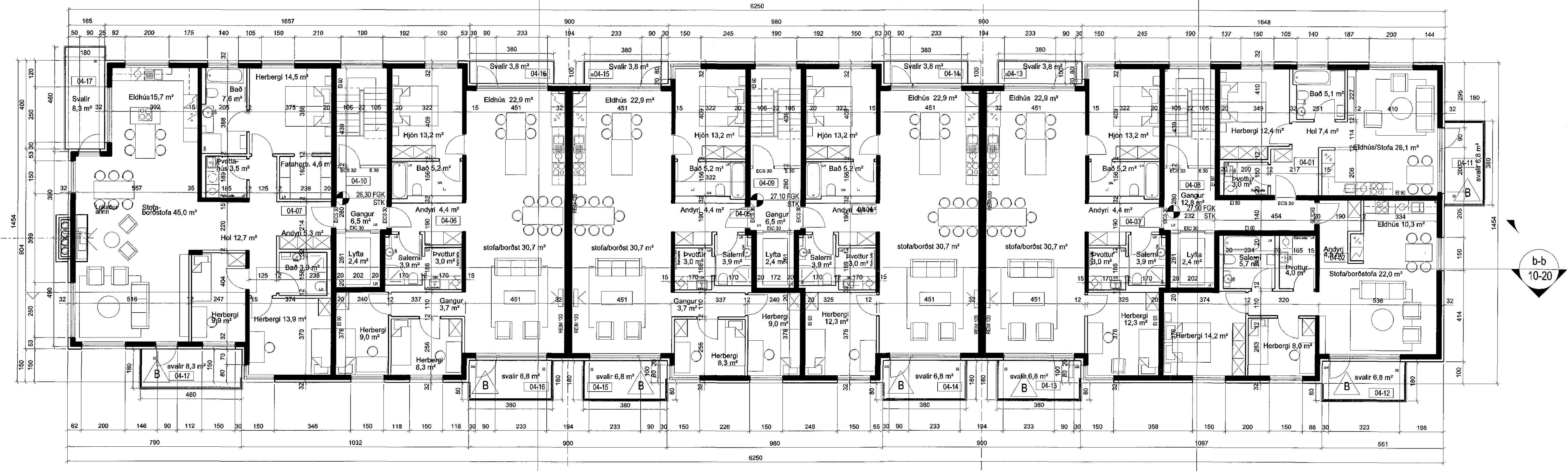
GRUNNMYND 4. HÆÐ 1:100
