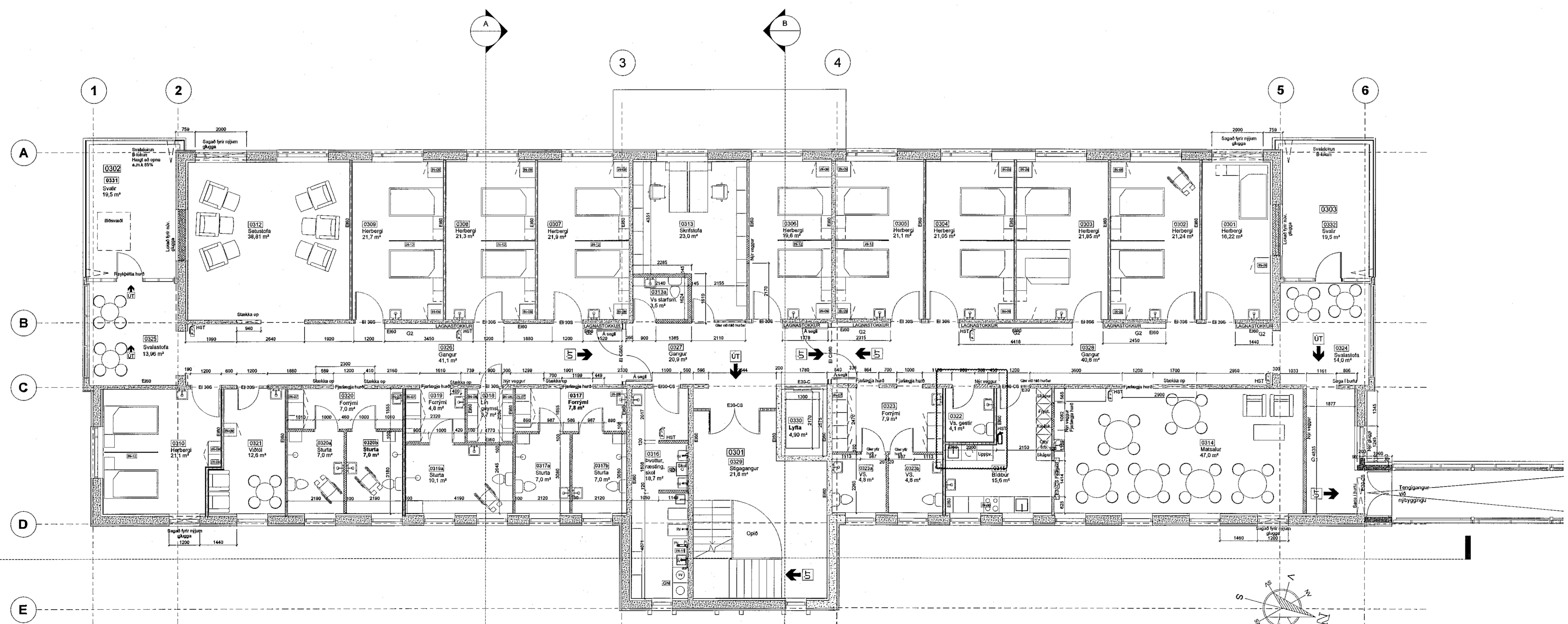
GRUNNMYND 2. HÆÐAR
