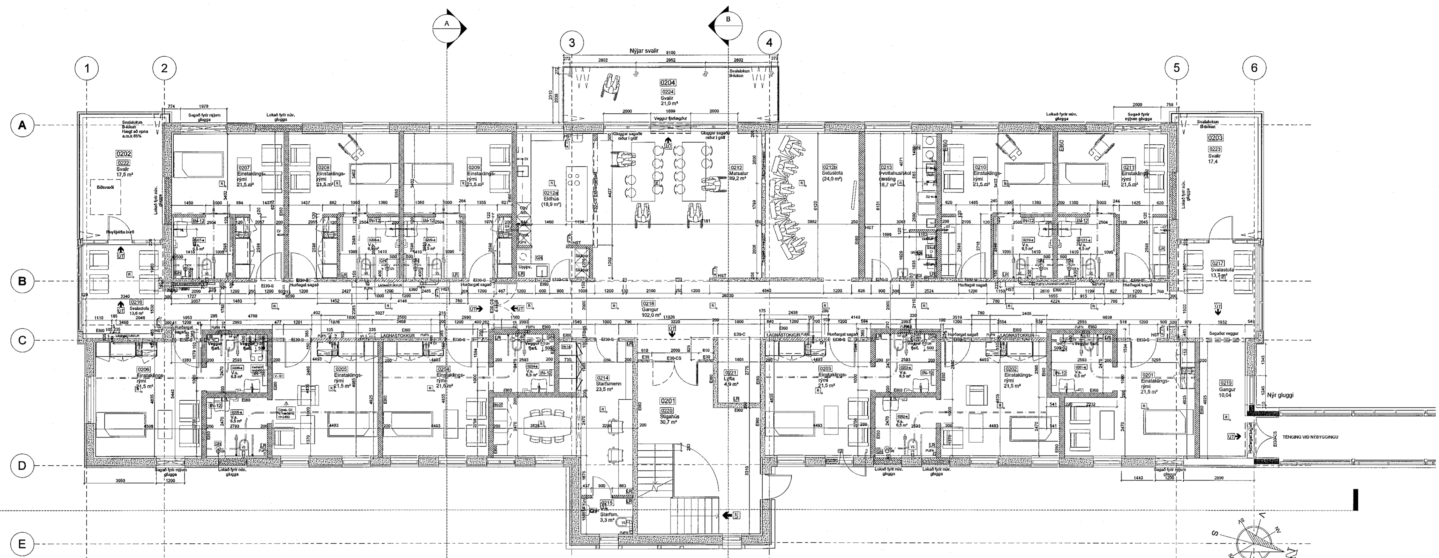
GRUNNMYND 2. HÆÐAR
