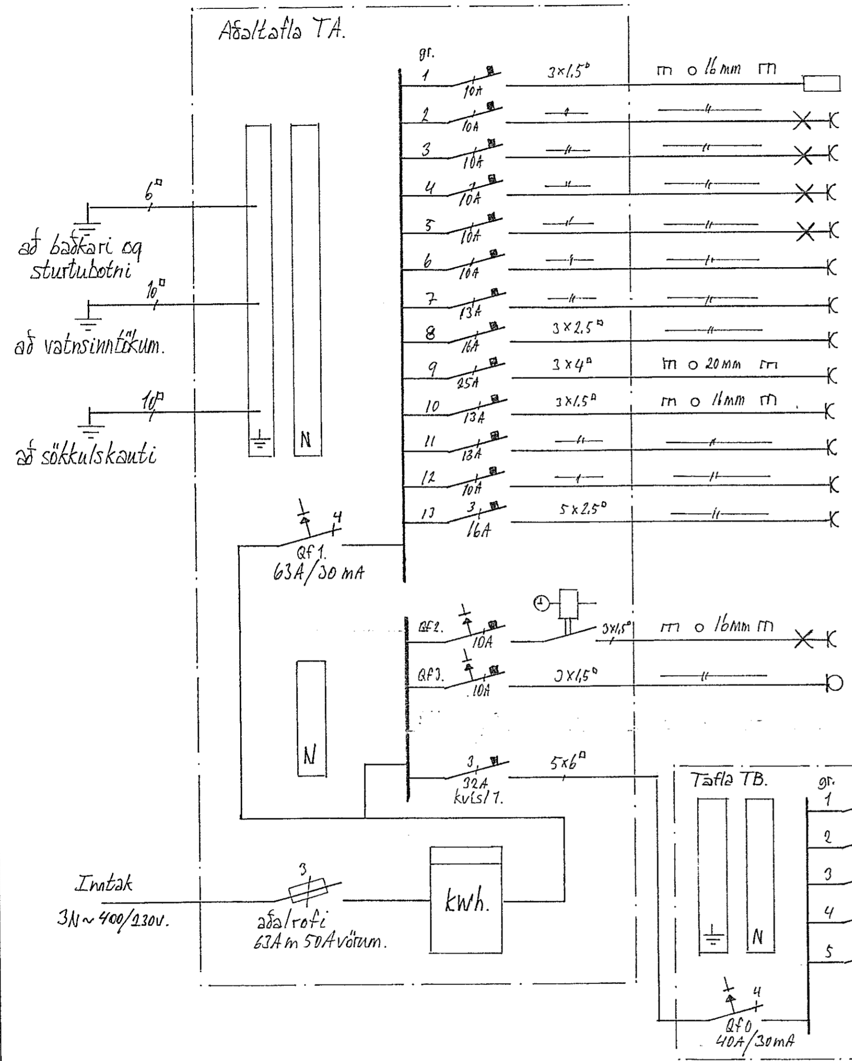
einlinamynd.
