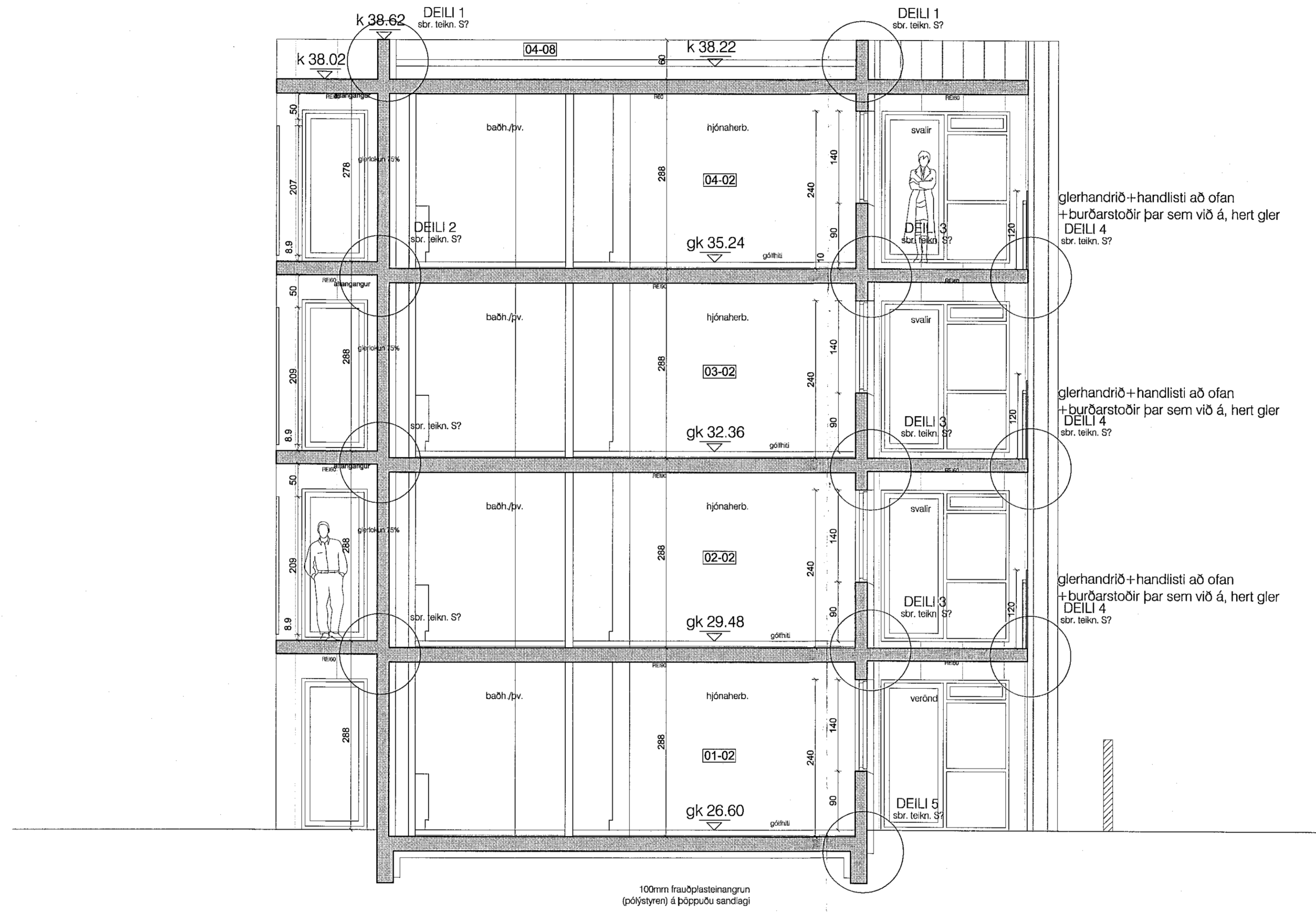
snið C-C
