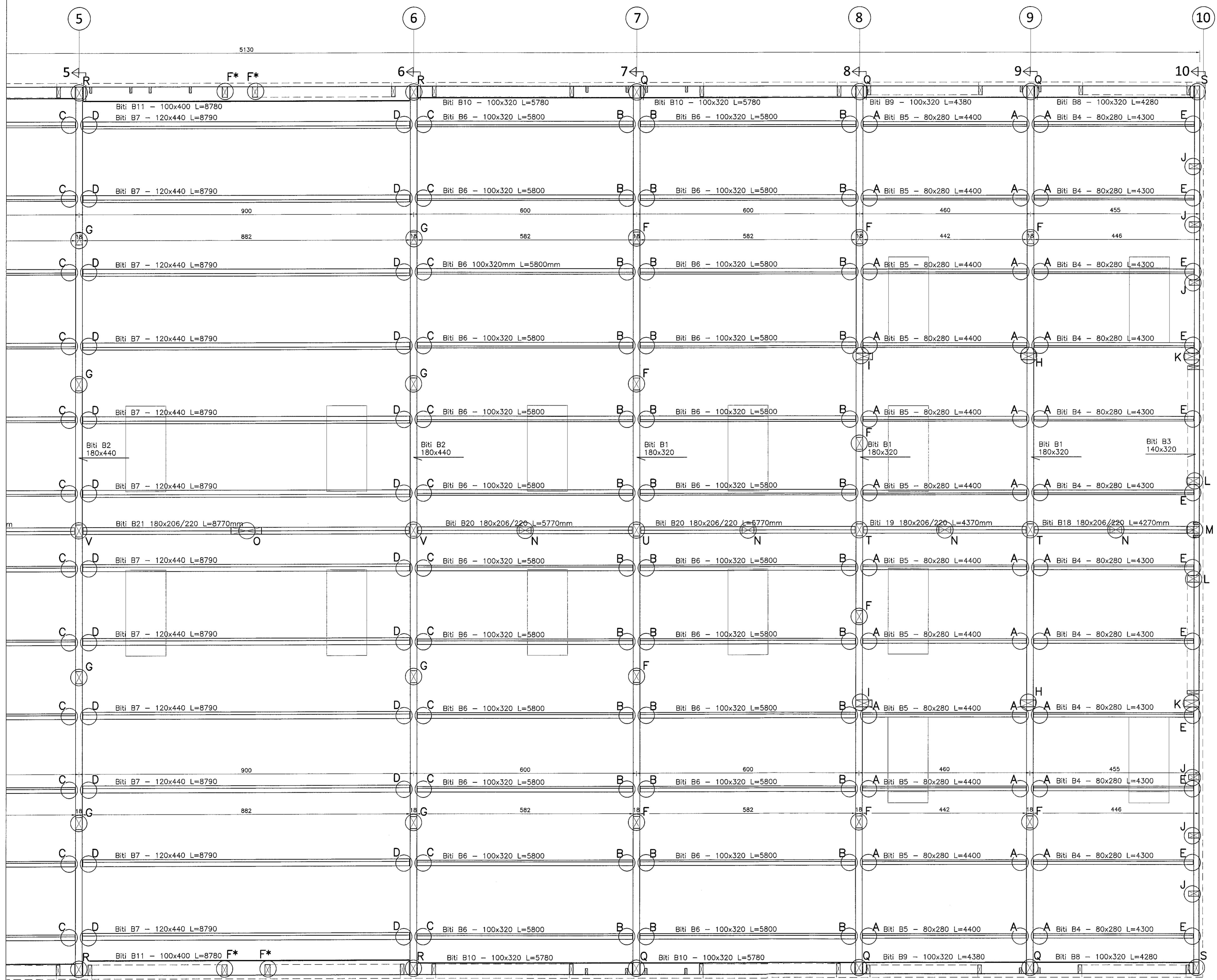
Grunnmynd þakviða (milli lína 5-10) 1:50
