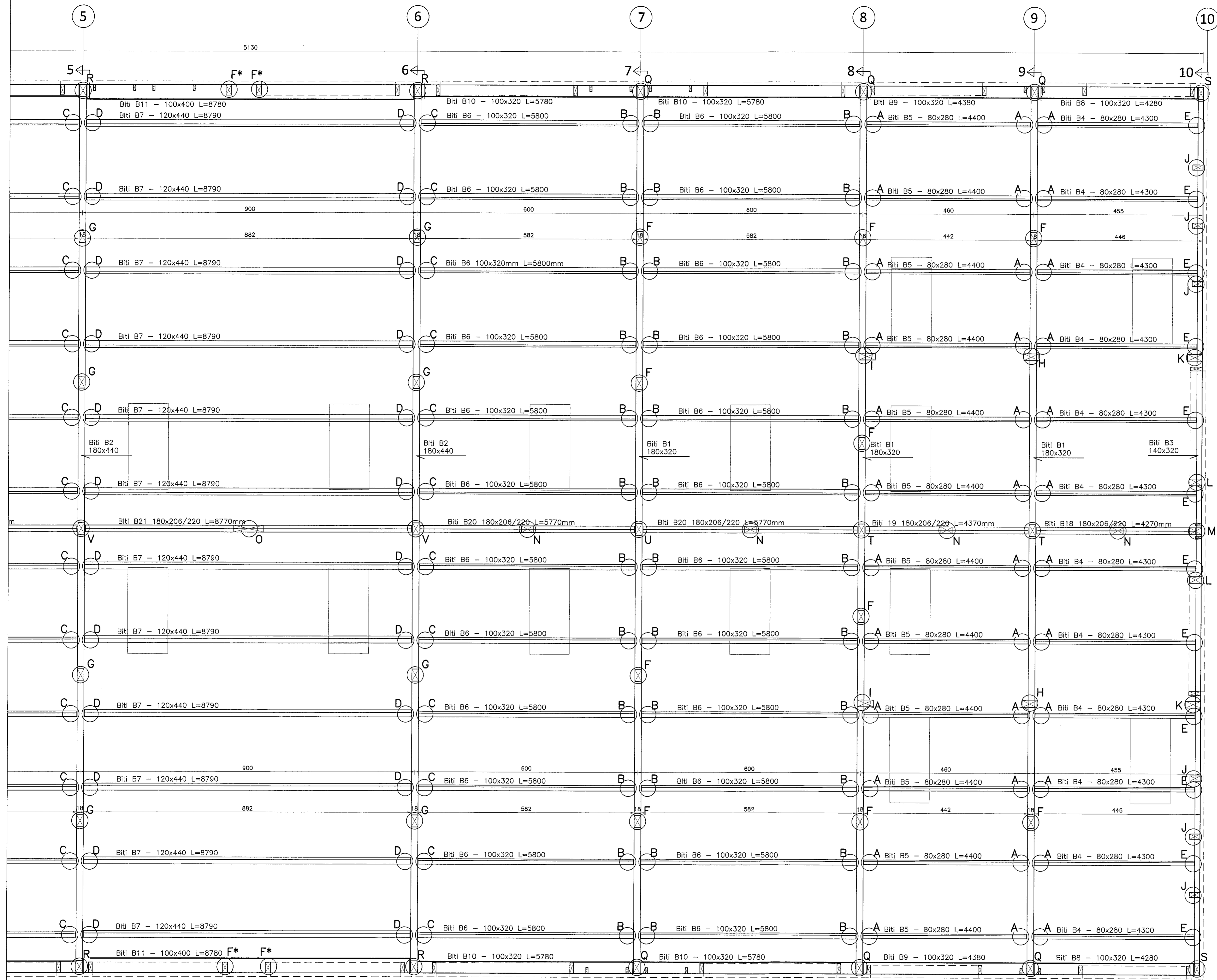
Grunnmýnd þakviða (milli lína 5-10) 1:50
